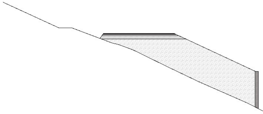
4 Profil 4 A00 1:100
