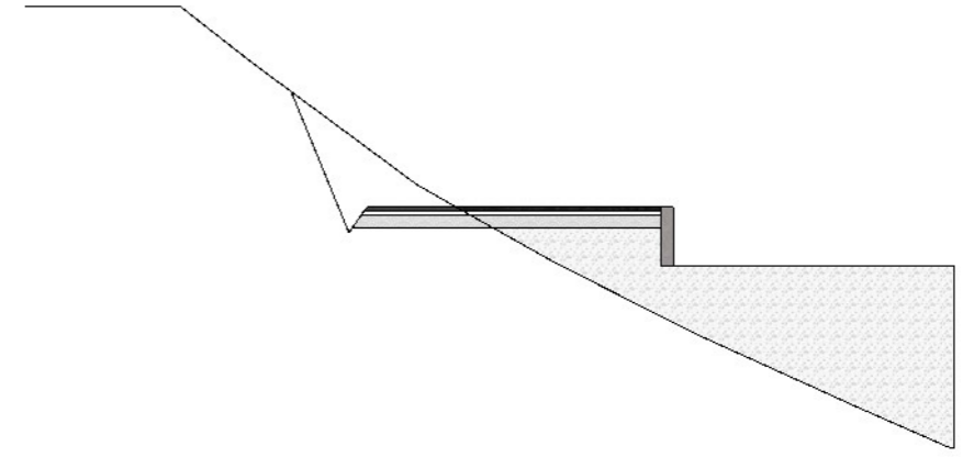
6 Profil 6 A00 1:100
