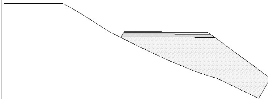
2 Profil 2 A00 1:100
