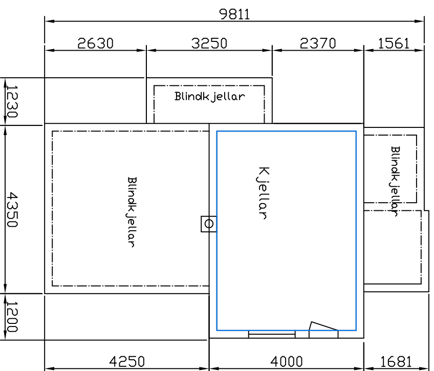
BRA 19 m 2 Kjellarplan
