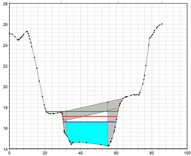
Figur 3-5 Geometri for oppstrøms bro sett fra oppstrøms side. Inkludert vannstand for de ulike vannførings scenarier. Blå: Q20, rød: Q200, grønn: Q200+20%
