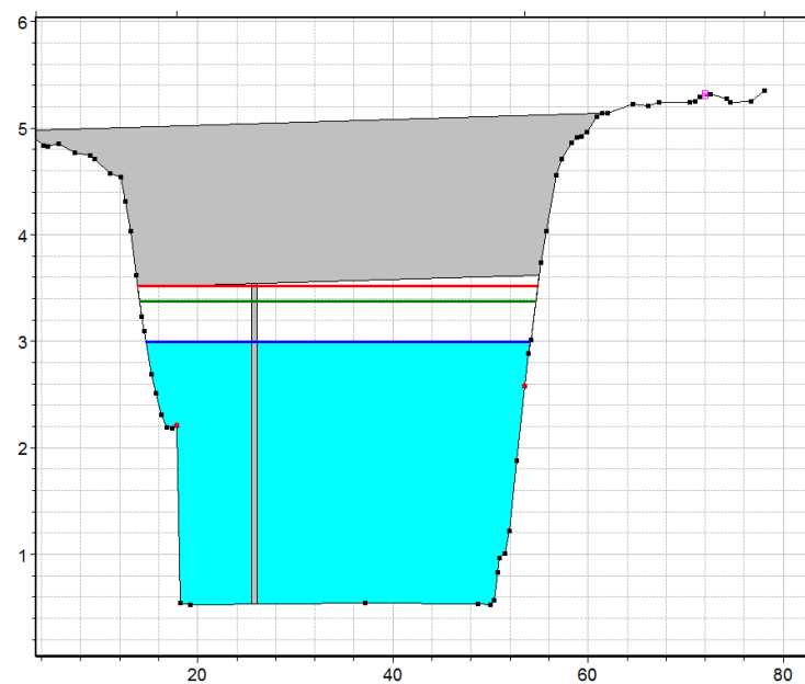
Figur 3-6 Geometri for nedstrøms bro sett fra oppstrøms side. Inkludert vannstand for de ulike vannførings scenarier. Blå: Q20, rød: Q200, grønn: Q200+20%
