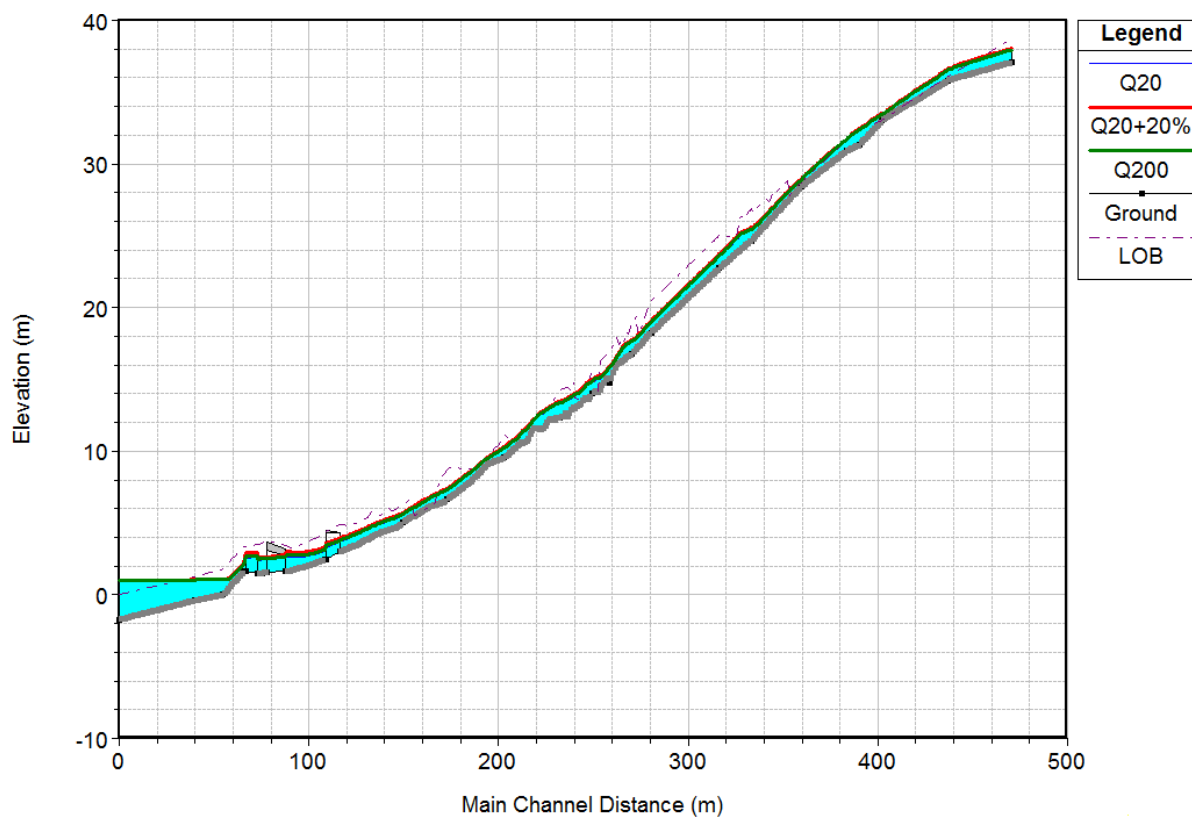
Figur 5-1 Simulerte vannstander for elv i Urdalen. Lengdeprofil
