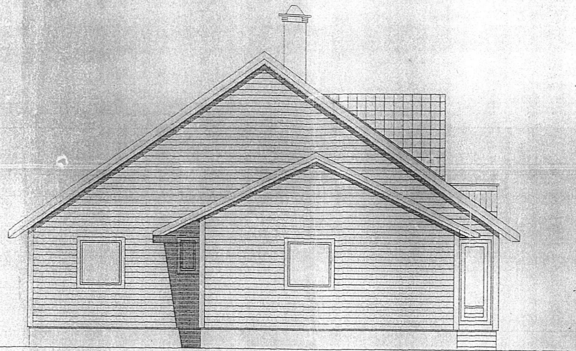
FASADE MOT NØR VEST
