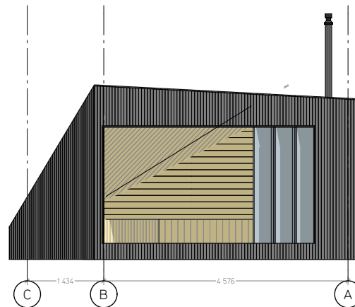
1:100 Fasade vest
