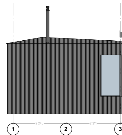
1:100 Fasade øst
