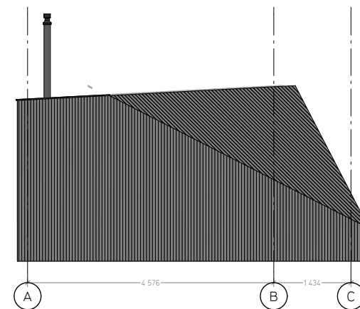
1:100 Fasade syd
