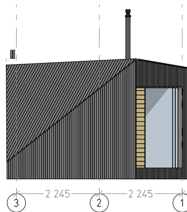
1:100 Fasade nord
