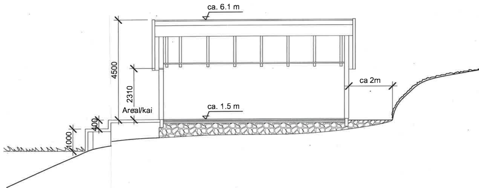
SNITT A-A
