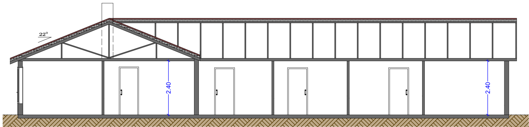
Snitt A-A
