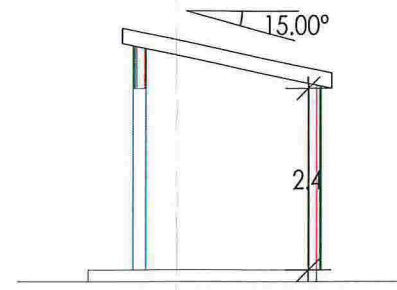
Snitt A-A
