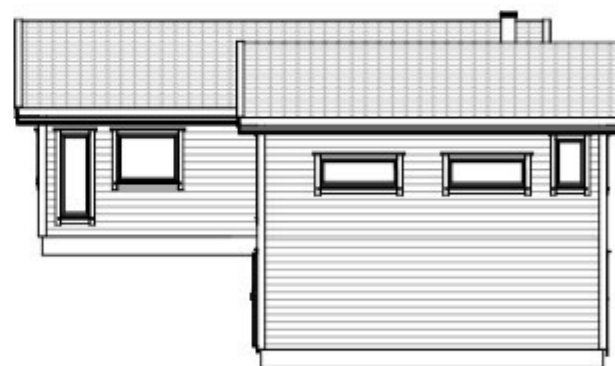
FASADE 4 1 : 100
