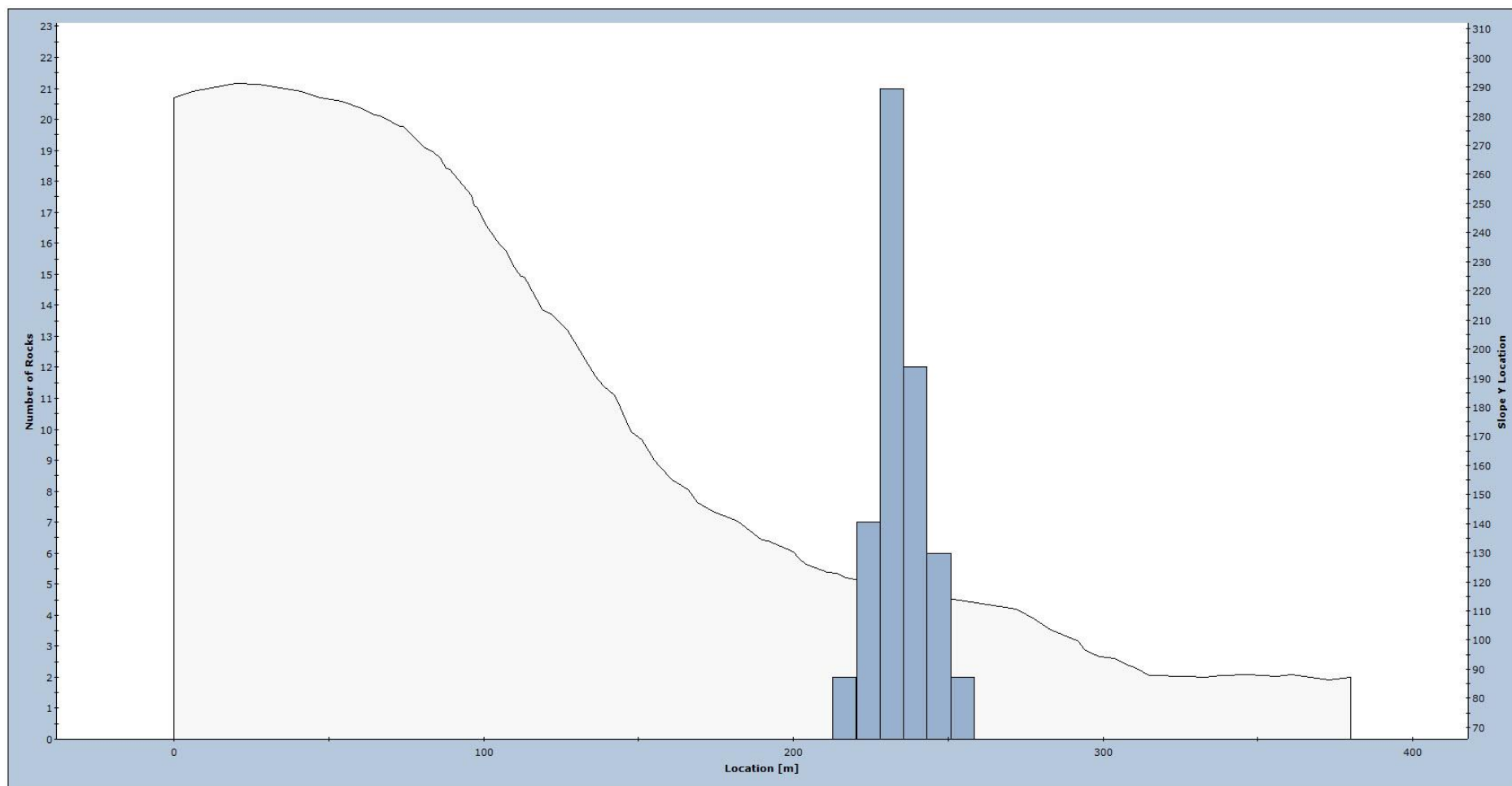
Figur 12. Fordeling av utløpsdistanser for modellerte steinsprang langs profil 1Krakeli.
