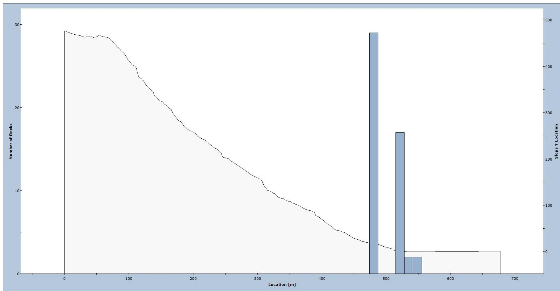
Figur 6. Fordeling av utløpsdistanser for modellerte steinsprang langs profil 1.
