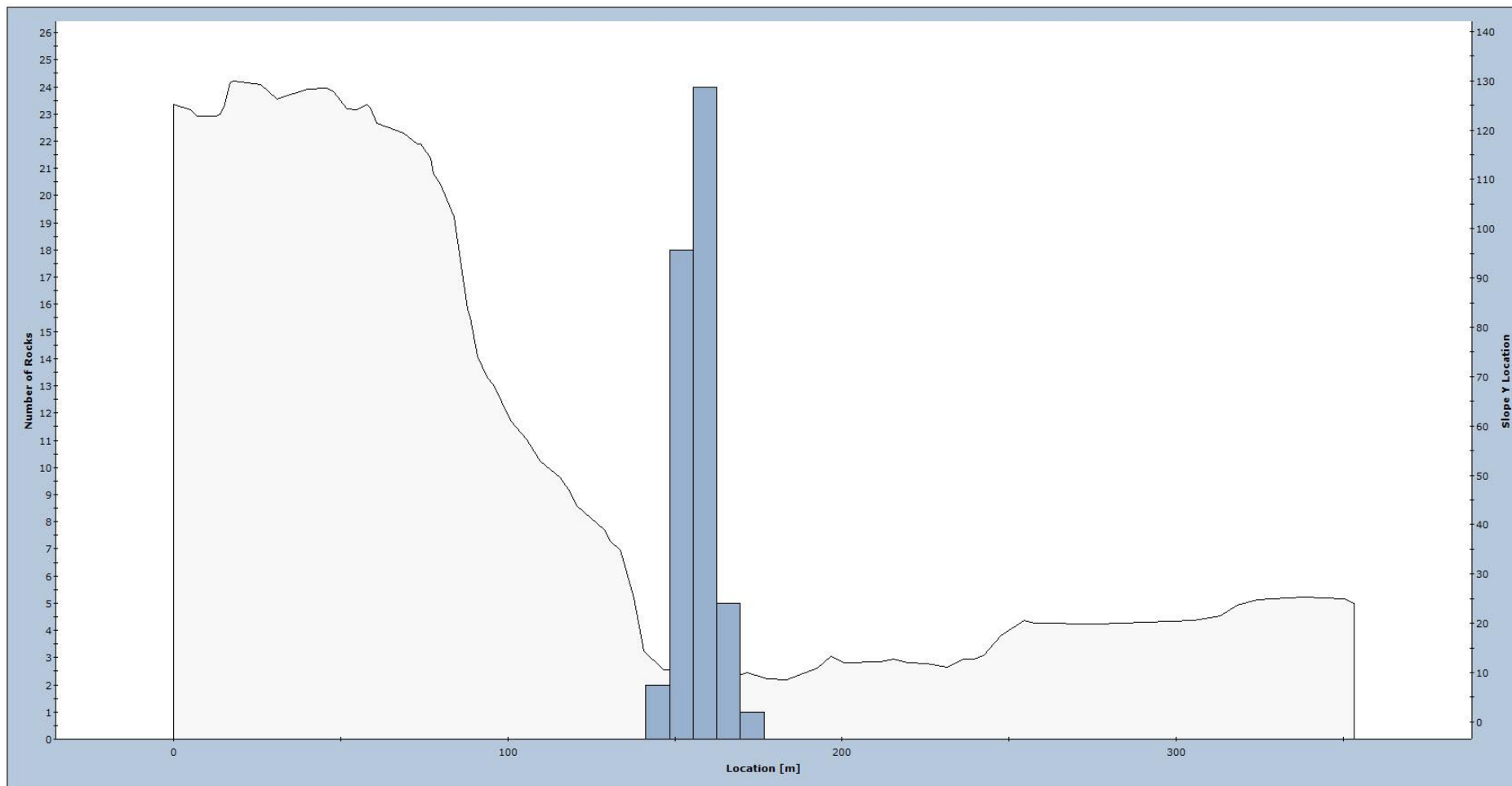
Figur 18. Fordeling av utløpsdistanser for modellerte steinsprang langs profil 1Havnfjellet.
