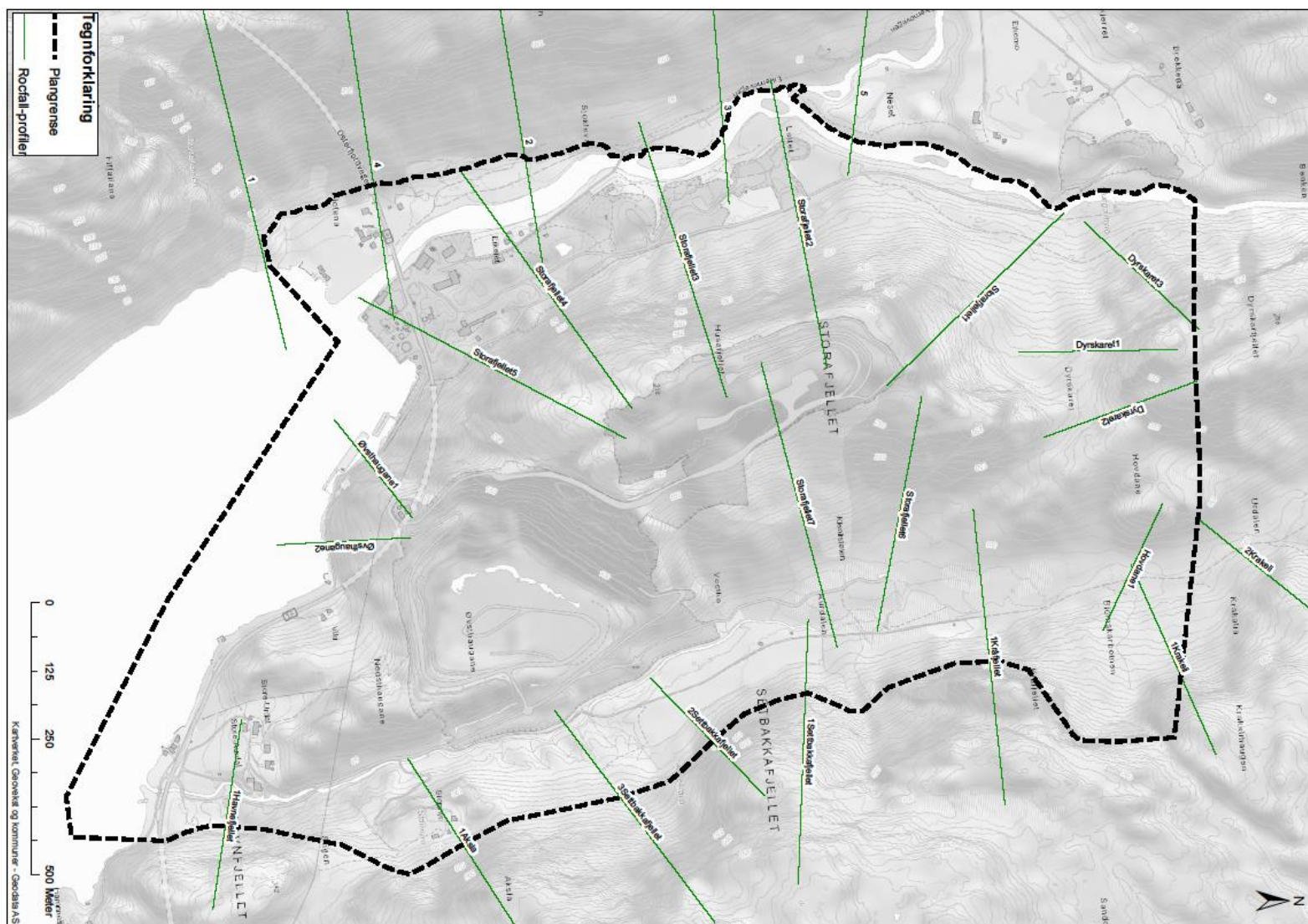
Figur 5. Lokasjon av de utvalgte terrengprofilene i planområdet. Se også tilhørende grafer med utløpsdistanser for steinsprang under.
