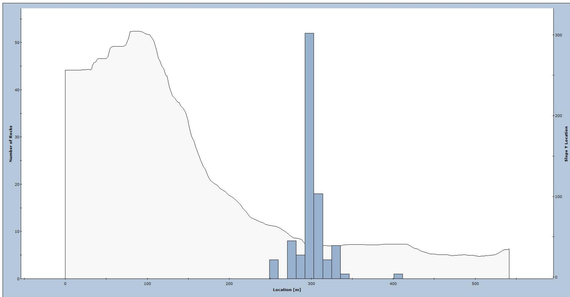
Figur 24. Fordeling av utløpsdistanser for modellerte steinsprang langs profil Storafjellet2.
