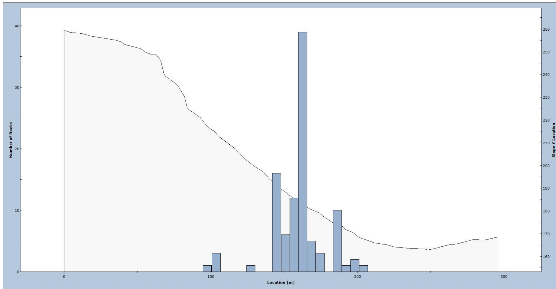
Figur 20. Fordeling av utløpsdistanser for modellerte steinsprang langs profil 2Dyrskaret.
