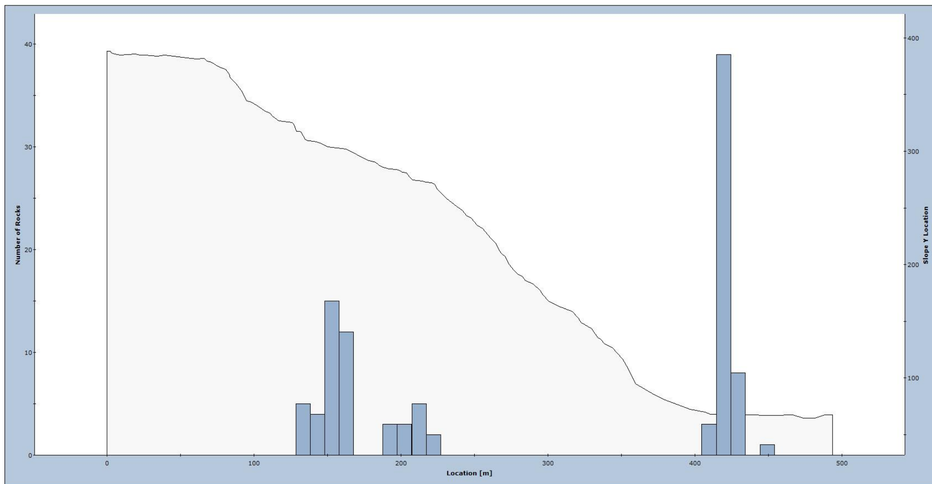
Figur 15. Fordeling av utløpsdistanser for modellerte steinsprang langs profil 1Settbakkafjellet.
