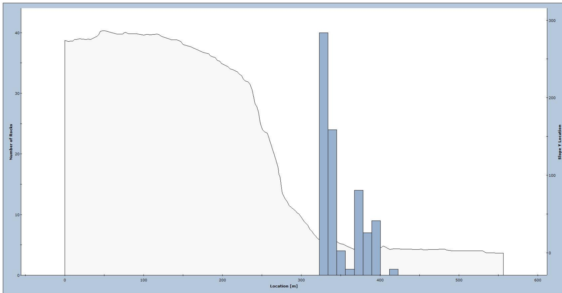
Figur 27. Fordeling av utløpsdistanser for modellerte steinsprang langs profil Storafjellet5.
