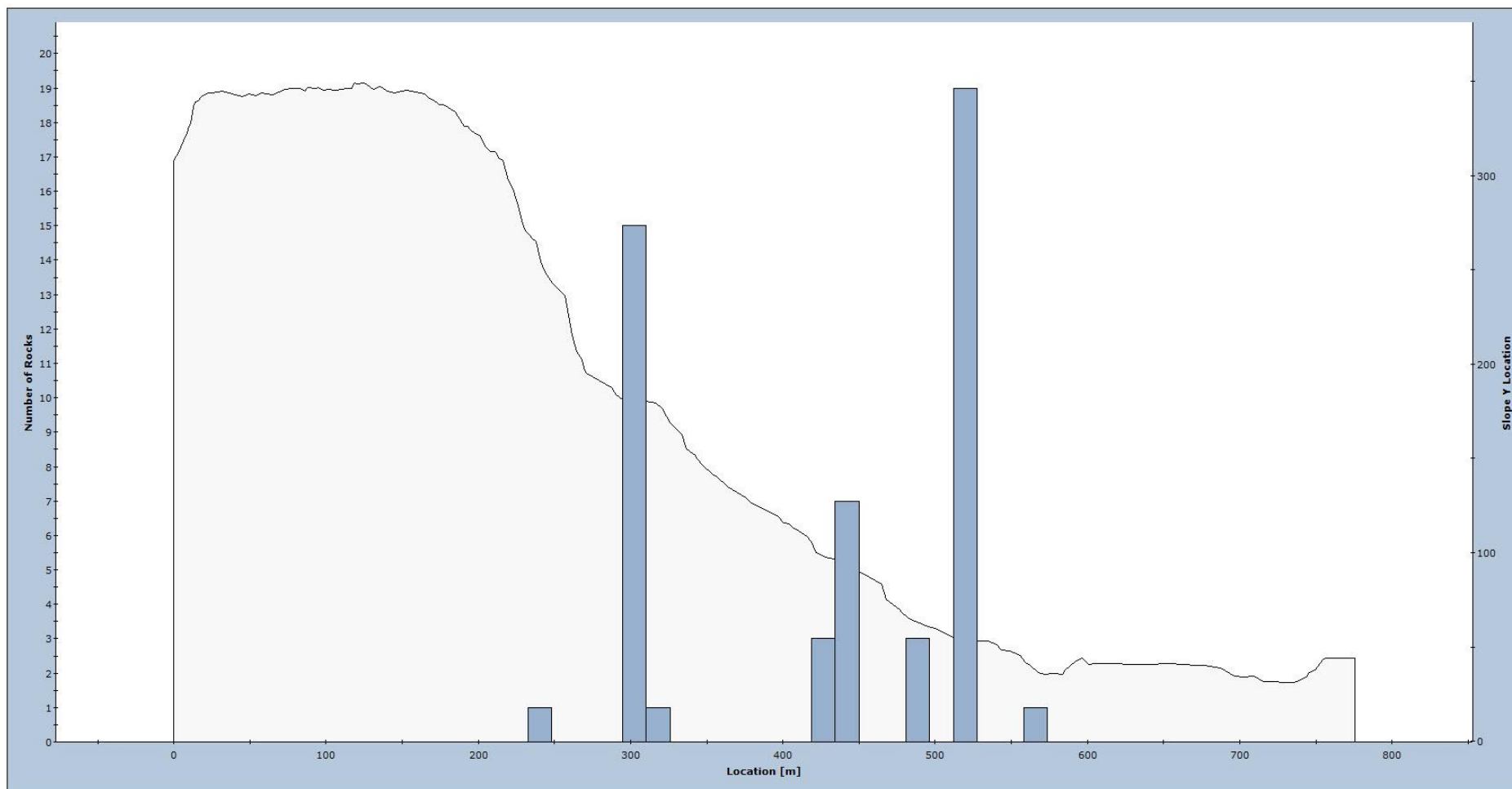
Figur 10. Fordeling av utløpsdistanser for modellerte steinsprang langs profil 5.
