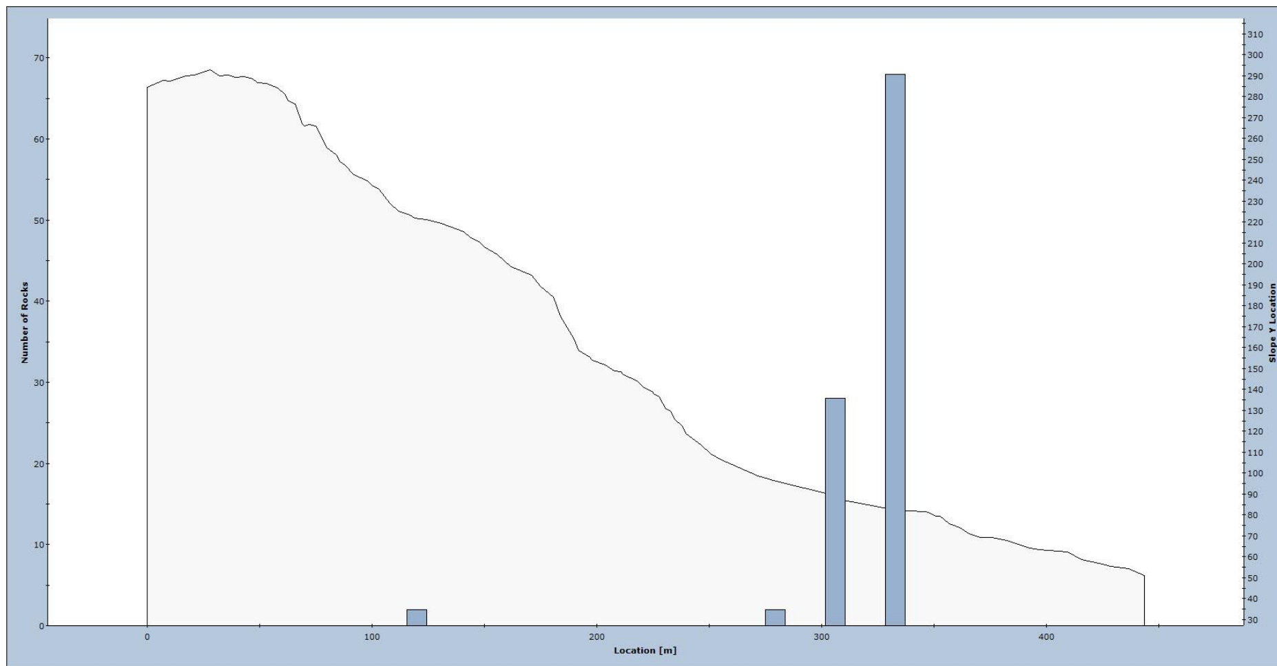
Figur 23. Fordeling av utløpsdistanser for modellerte steinsprang langs profil Storafjellet1.
