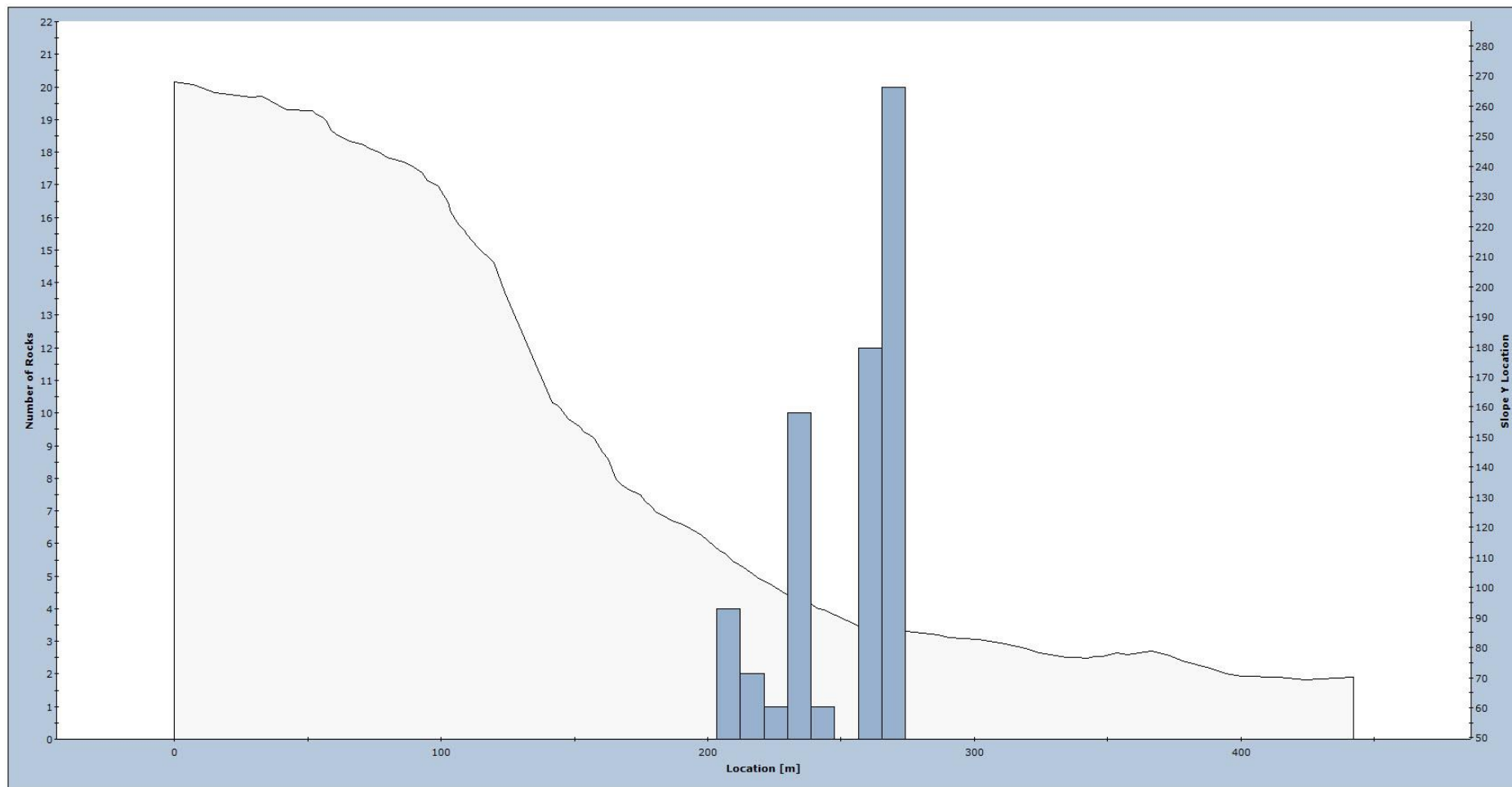
Figur 28. Fordeling av utløpsdistanser for modellerte steinsprang langs profil Storafjellet6.
