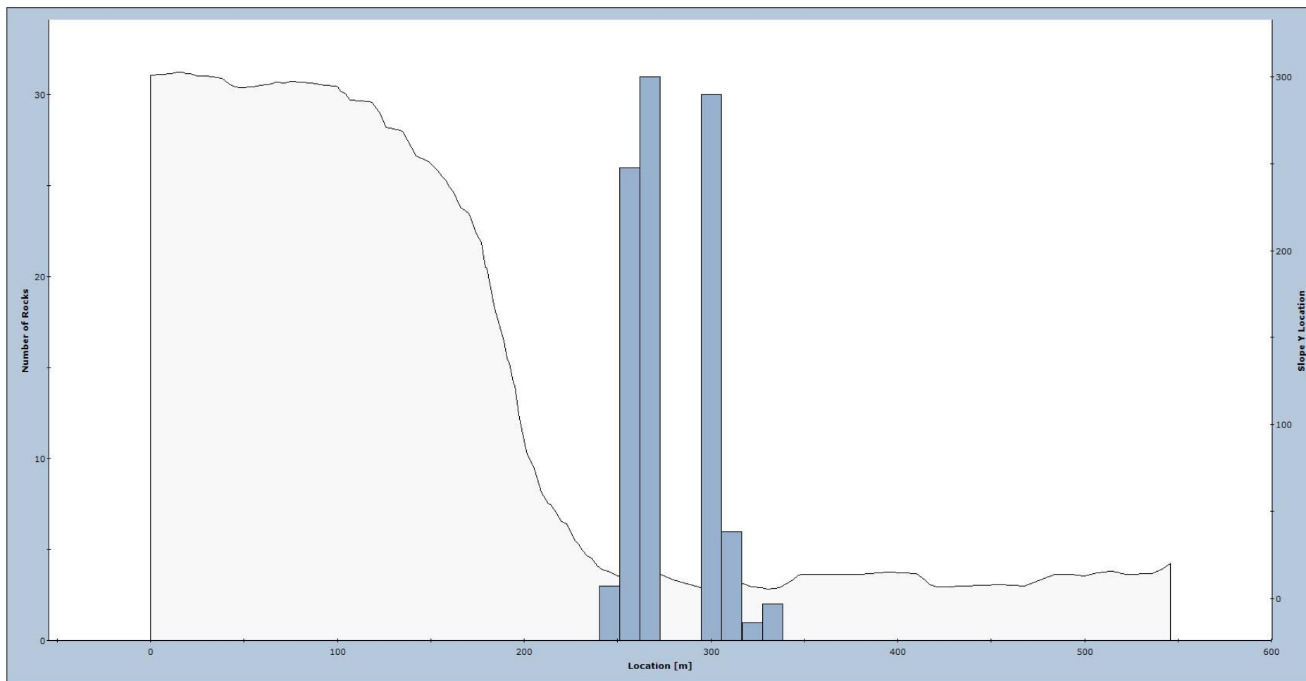
Figur 26. Fordeling av utløpsdistanser for modellerte steinsprang langs profil Storafjellet4.
