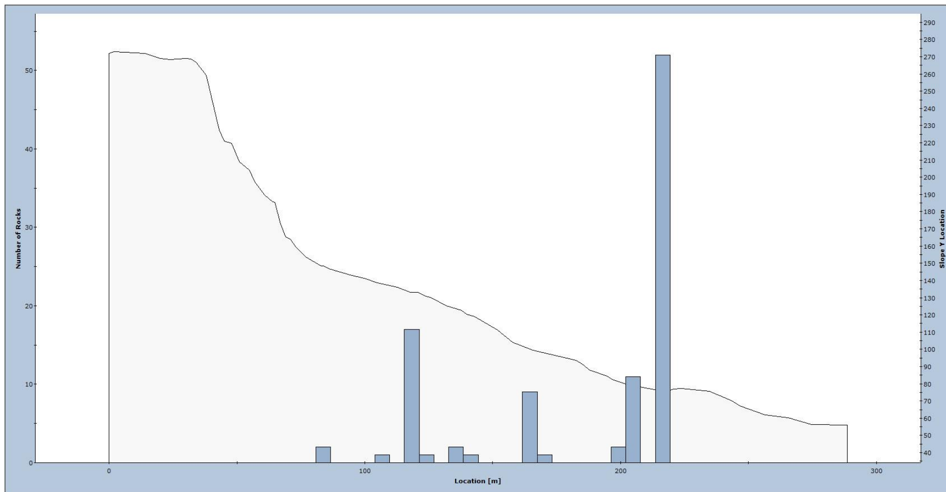
Figur 21. Fordeling av utløpsdistanser for modellerte steinsprang langs profil 3Dyrskaret.
