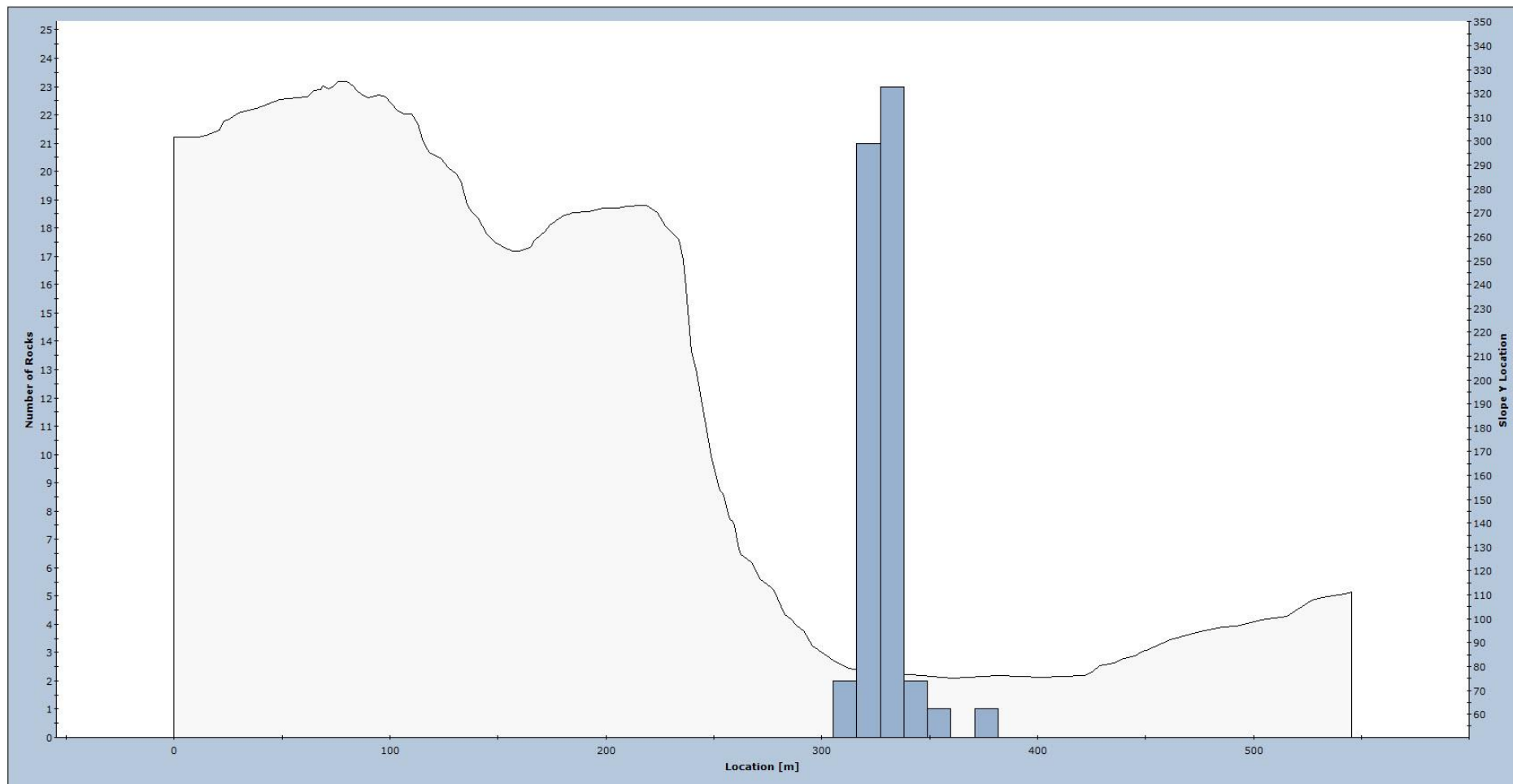
Figur 14. Fordeling av utløpsdistanser for modellerte steinsprang langs profil 1Kråfjellet.
