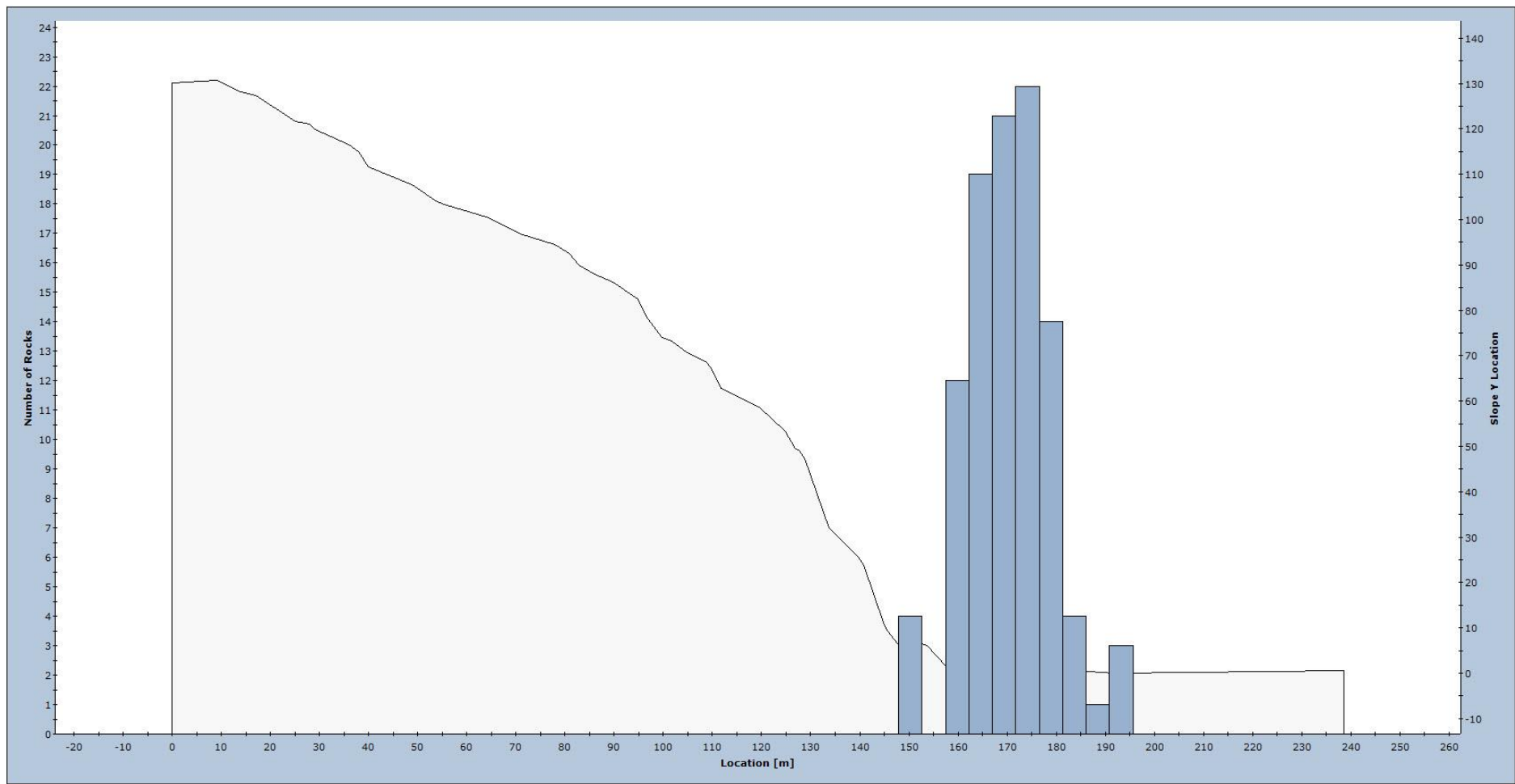
Figur 31. Fordeling av utløpsdistanser for modellerte steinsprang langs profil Øvsthaugane2.
