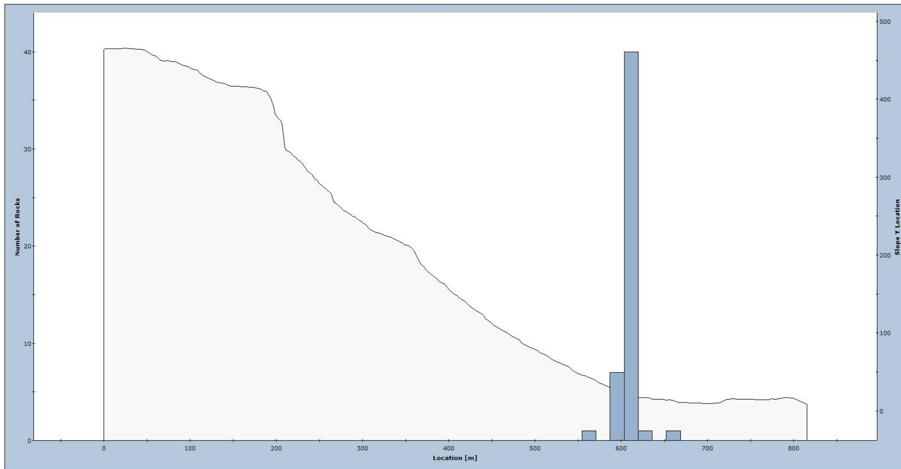
Figur 7. Fordeling av utløpsdistanser for modellerte steinsprang langs profil 2.
