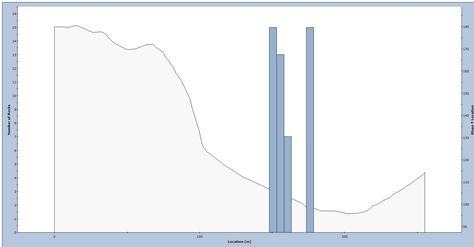
Figur 13. Fordeling av utløpsdistanser for modellerte steinsprang langs profil 2Krakeli.
