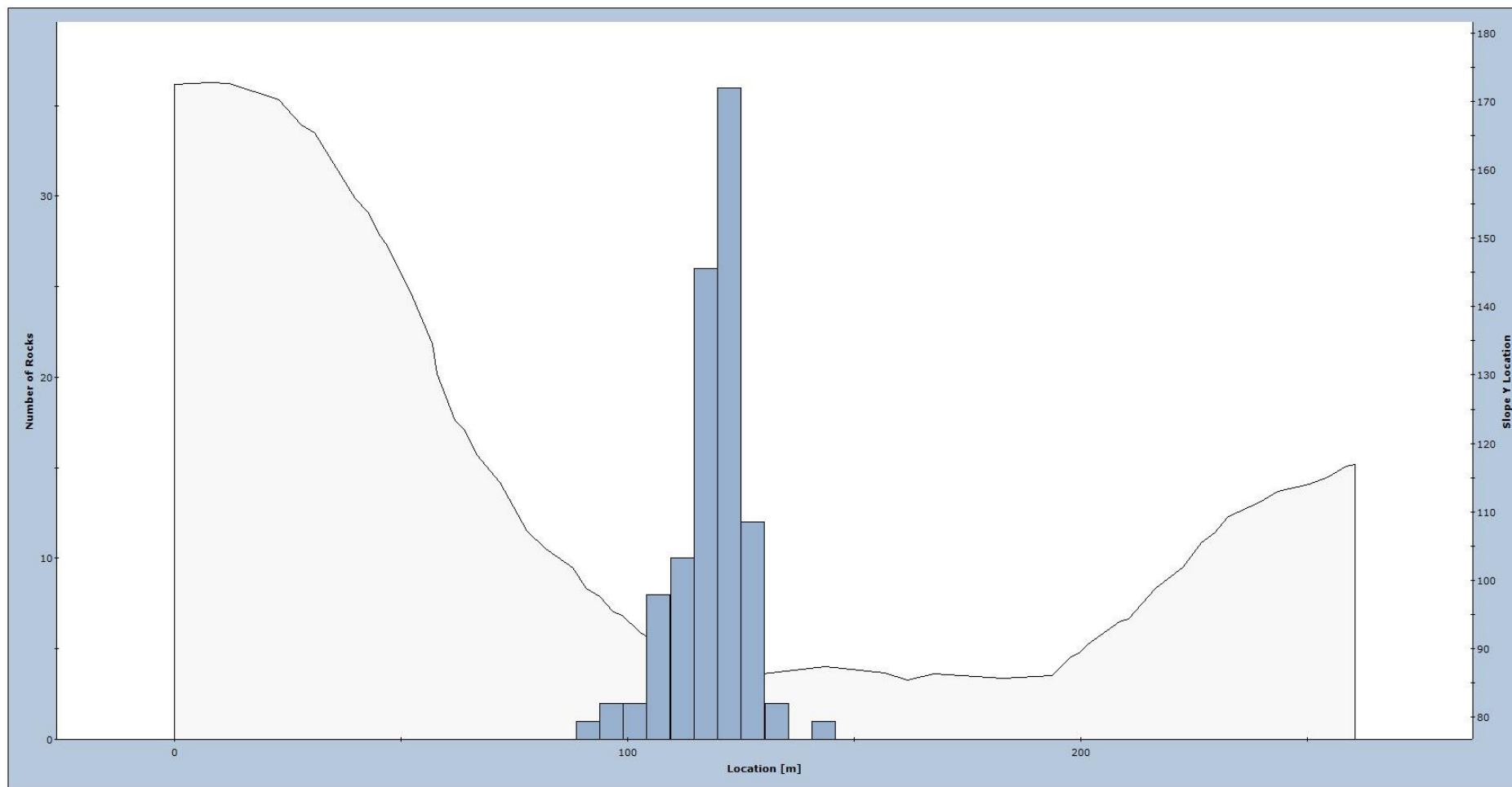
Figur 22. Fordeling av utløpsdistanser for modellerte steinsprang langs profil 1Hovdane.
