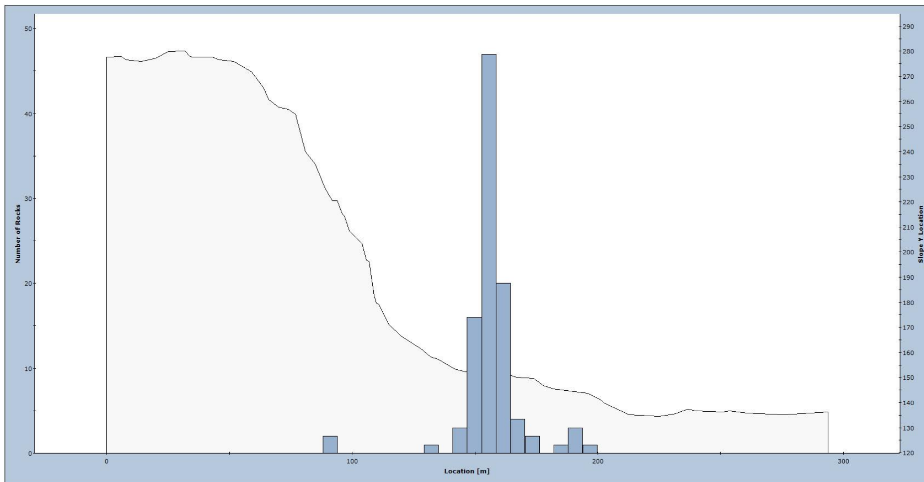
Figur 19. Fordeling av utløpsdistanser for modellerte steinsprang langs profil 1Dyrskaret.
