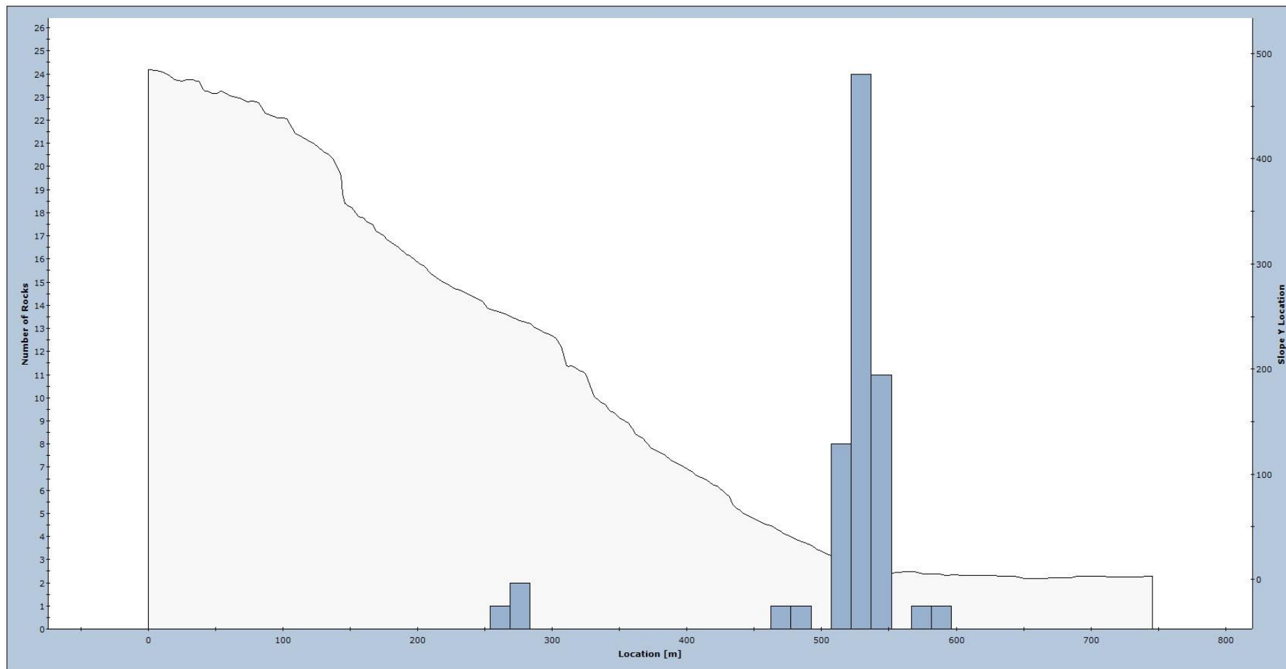
Figur 9. Fordeling av utløpsdistanser for modellerte steinsprang langs profil 4.
