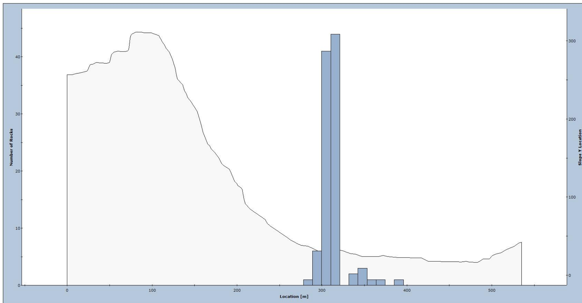
Figur 25. Fordeling av utløpsdistanser for modellerte steinsprang langs profil Storafjellet3.
