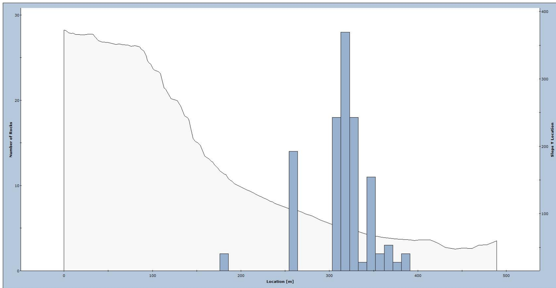
Figur 17. Fordeling av utløpsdistanser for modellerte steinsprang langs profil 3Settbakkafjellet.
