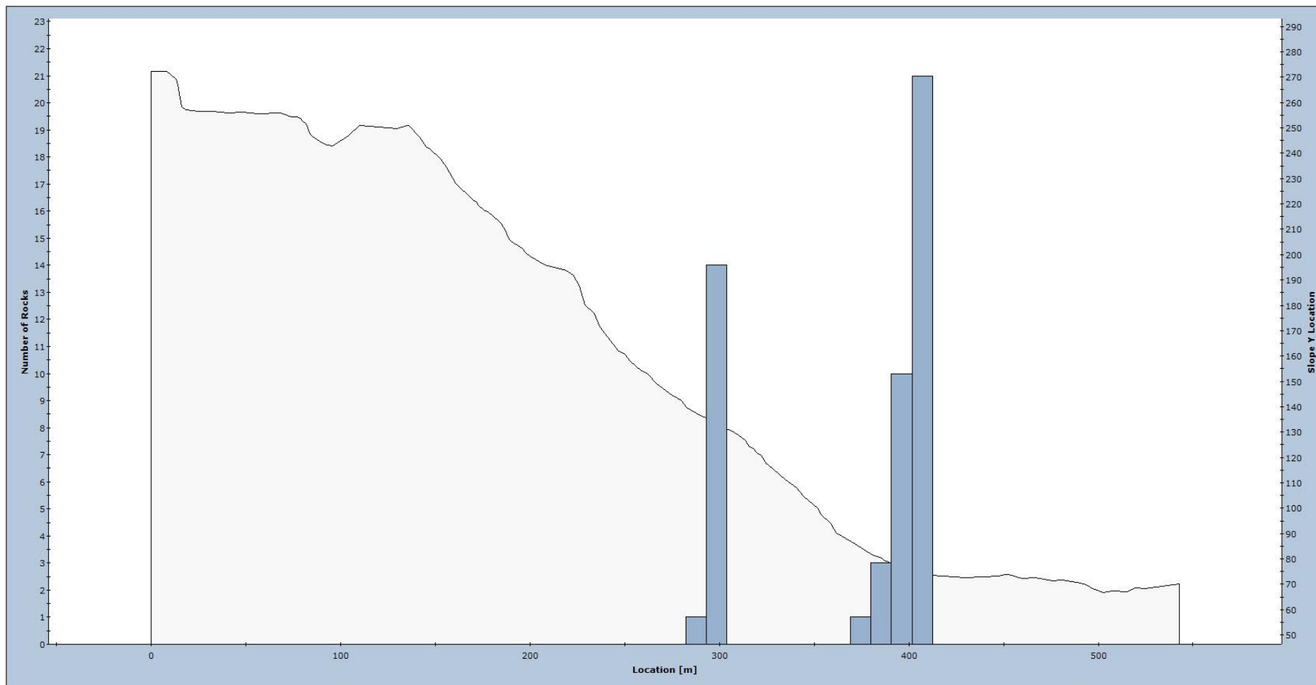
Figur 29. Fordeling av utløpsdistanser for modellerte steinsprang langs profil Storafjellet7.
