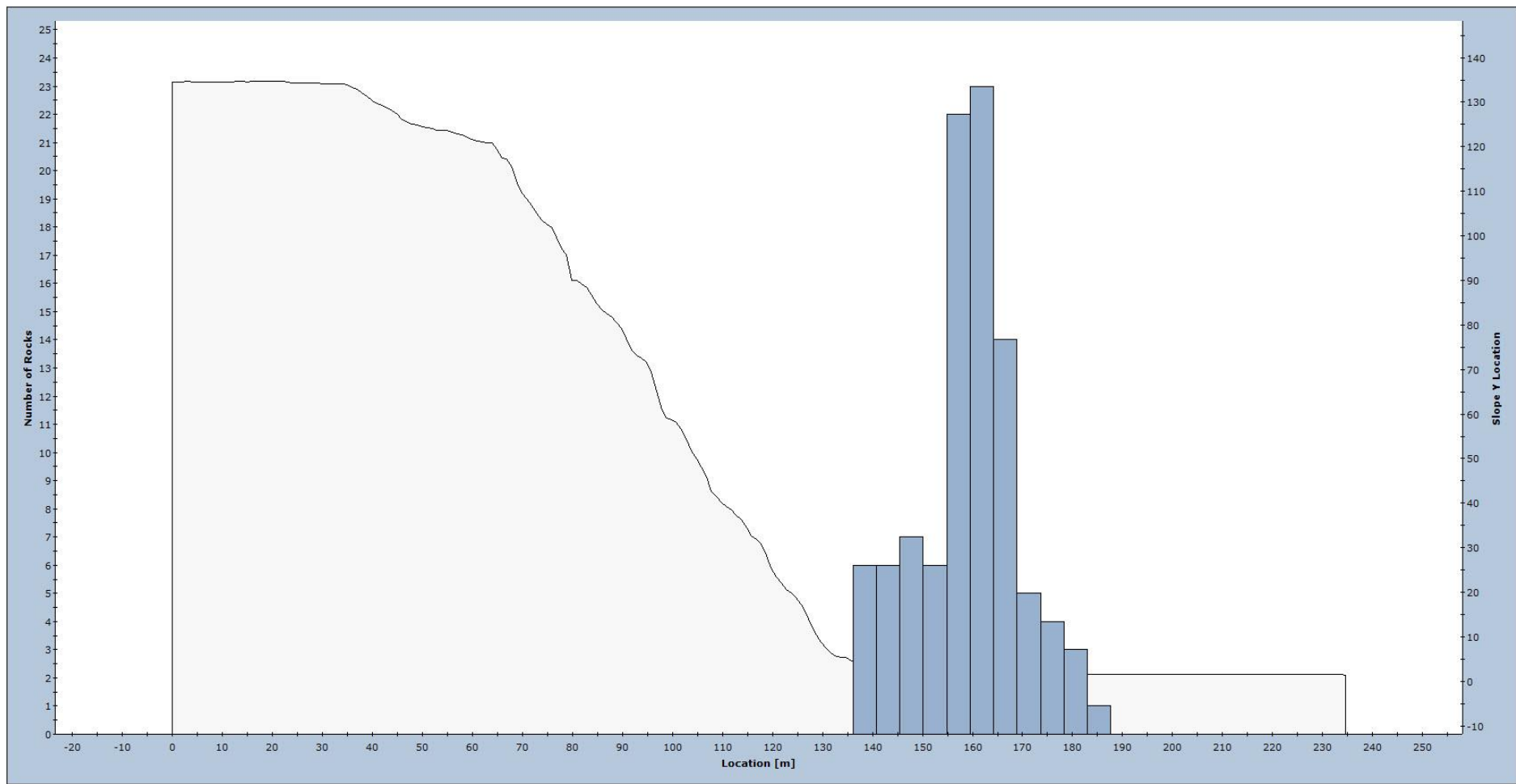
Figur 30. Fordeling av utløpsdistanser for modellerte steinsprang langs profil Øvsthaugane1.
