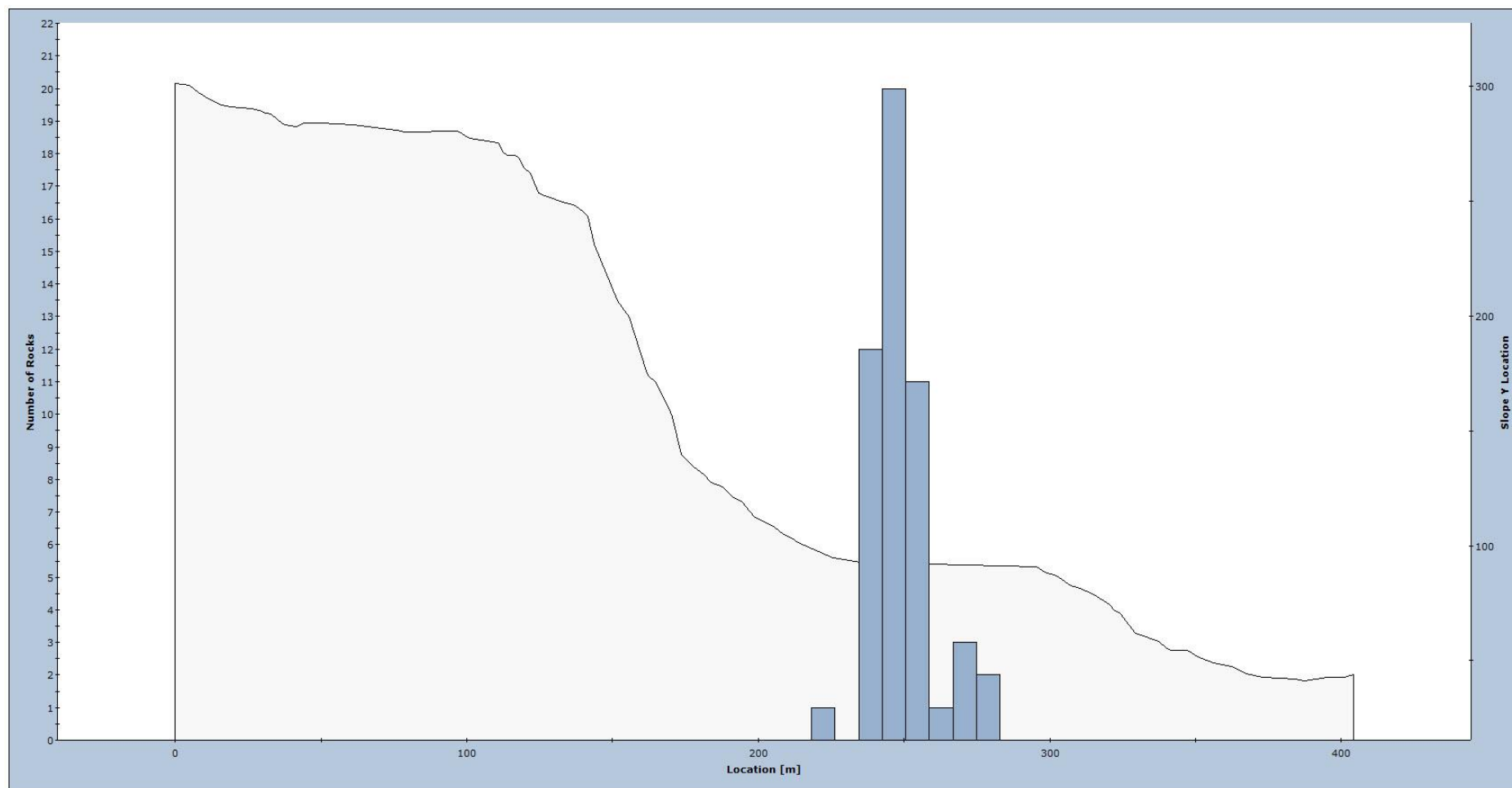
Figur 11. Fordeling av utløpsdistanser for modellerte steinsprang langs profil 1Aksla.
