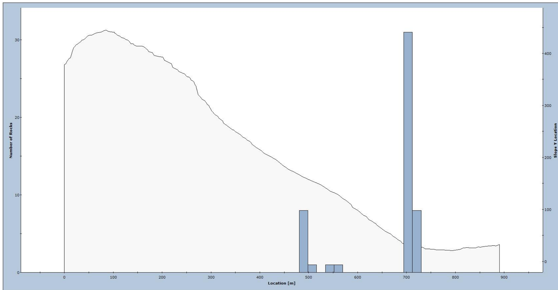
Figur 8. Fordeling av utløpsdistanser for modellerte steinsprang langs profil 3.
