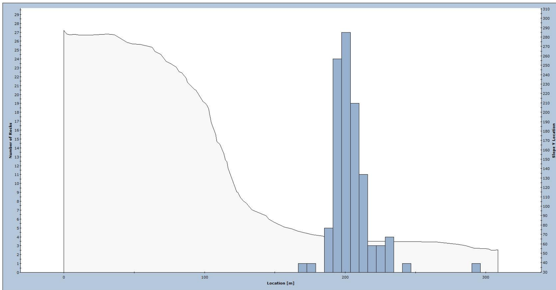
Figur 16. Fordeling av utløpsdistanser for modellerte steinsprang langs profil 2Settbakkafjellet.
