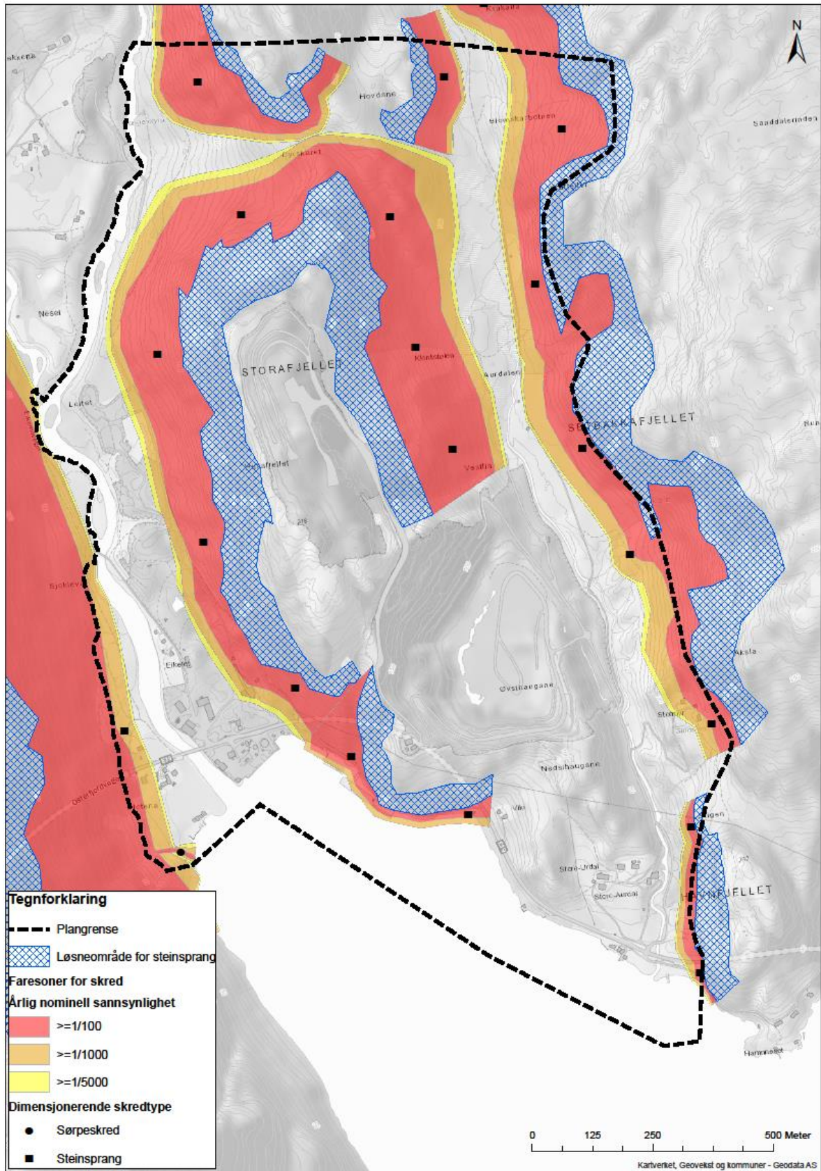
Figur 32. Faresonekart for steinsprang/-skred med faresonegrenser for årlig nominell sannsynlighet innenfor planområdet. Faresonegrensene er dimensjonert for steinsprang og sørpeskred fra naturlig terreng.
