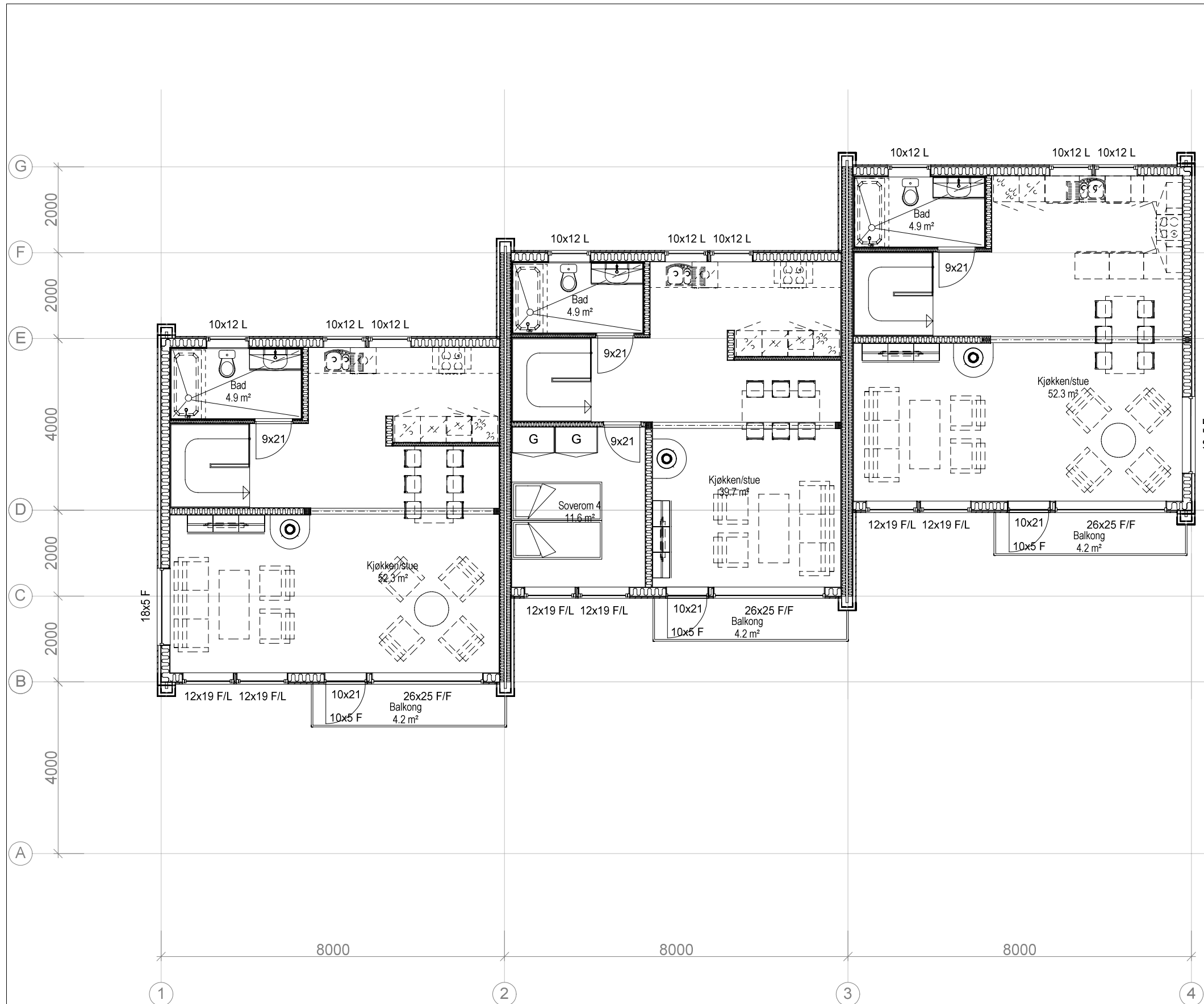
BOLIG 35 Plan 2. etasje BRA 58,1 m2
