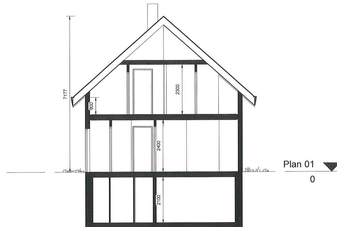
3 Snitt 2 1 : 100 Snitt - eksisterende bolig
