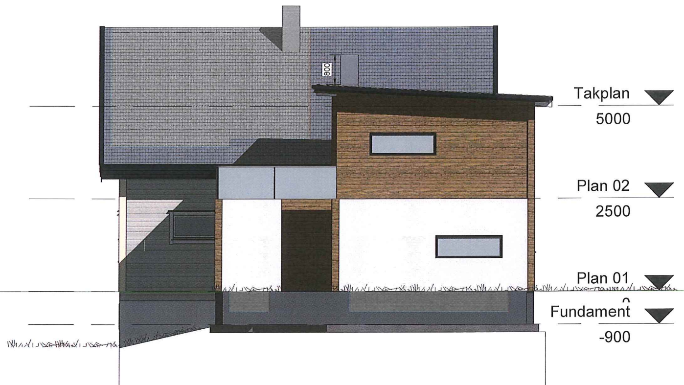
1 Vest 1 : 100
