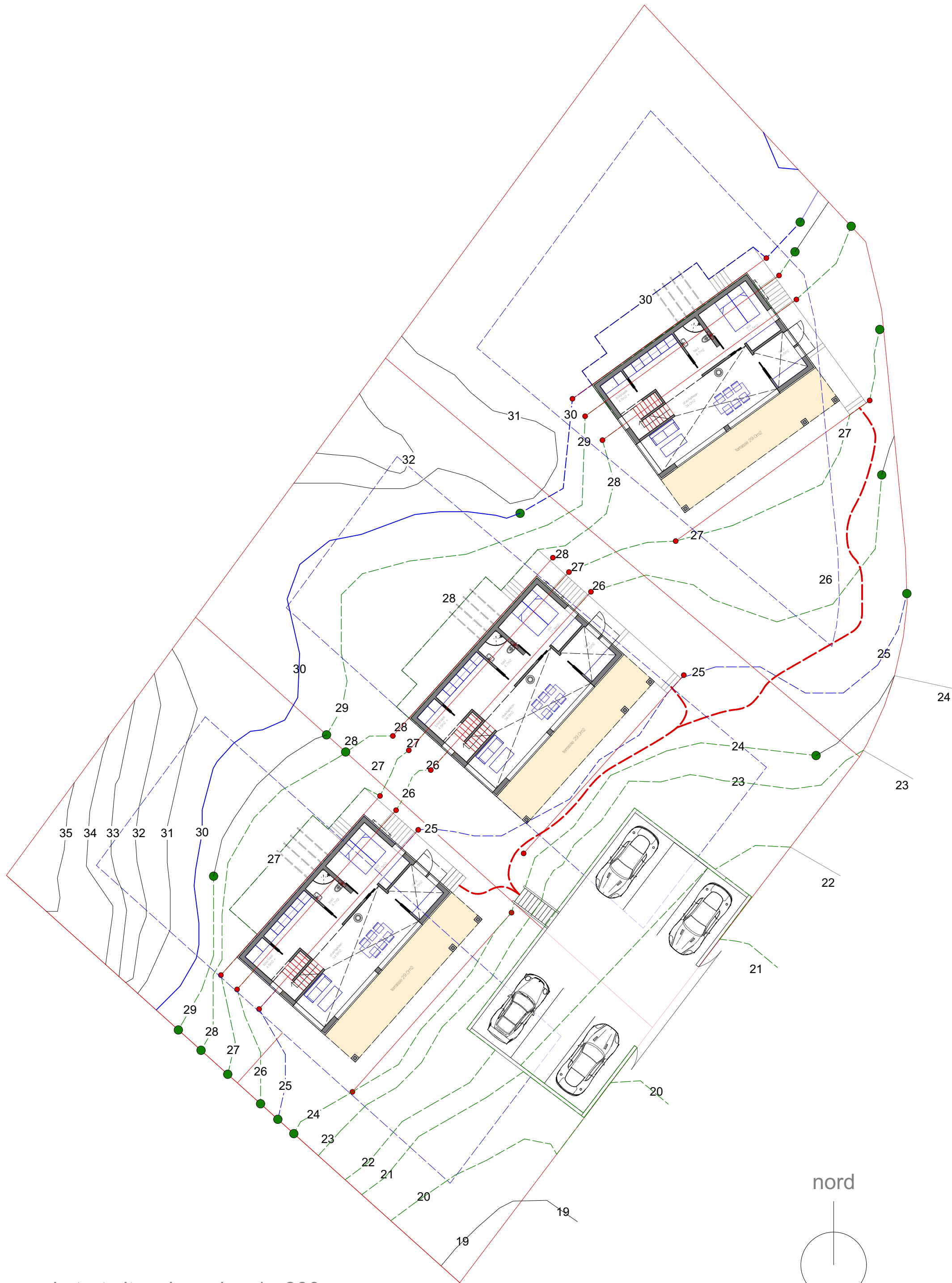
kotert situasjonsplan 1 : 200
