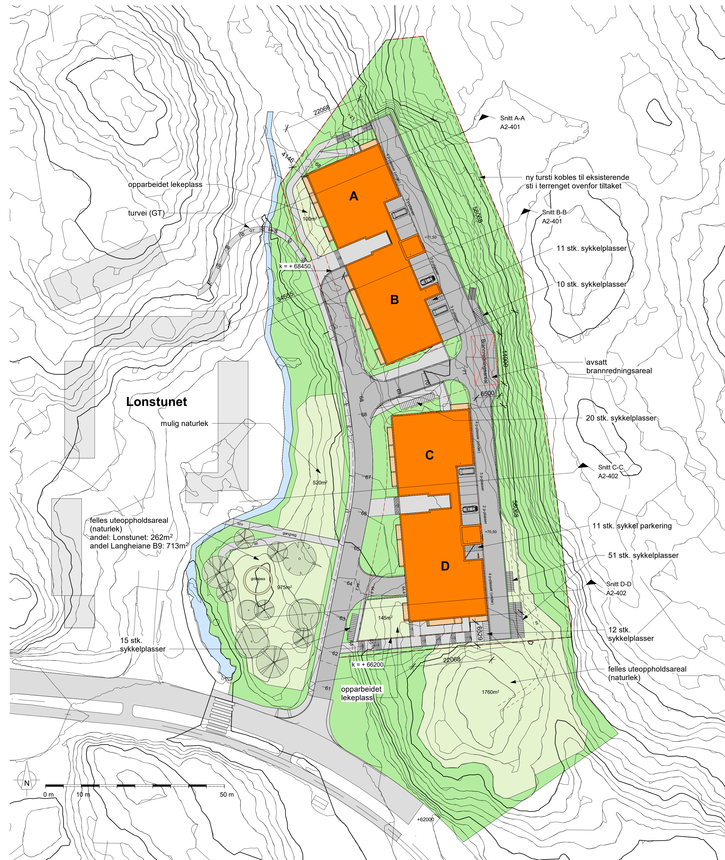
1 Situasjon 1 : 500
