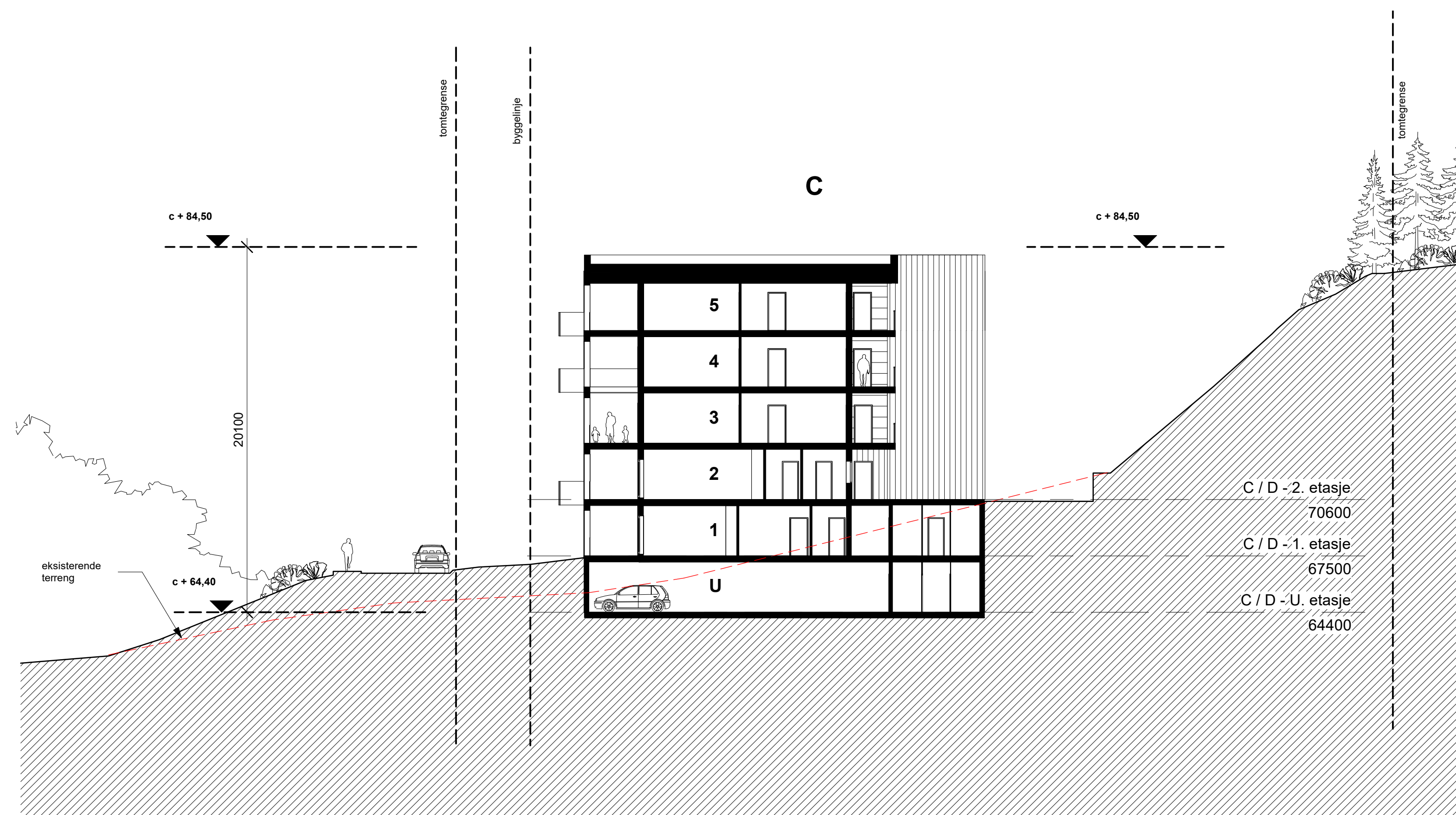
1 Snitt C-C 1 : 200
