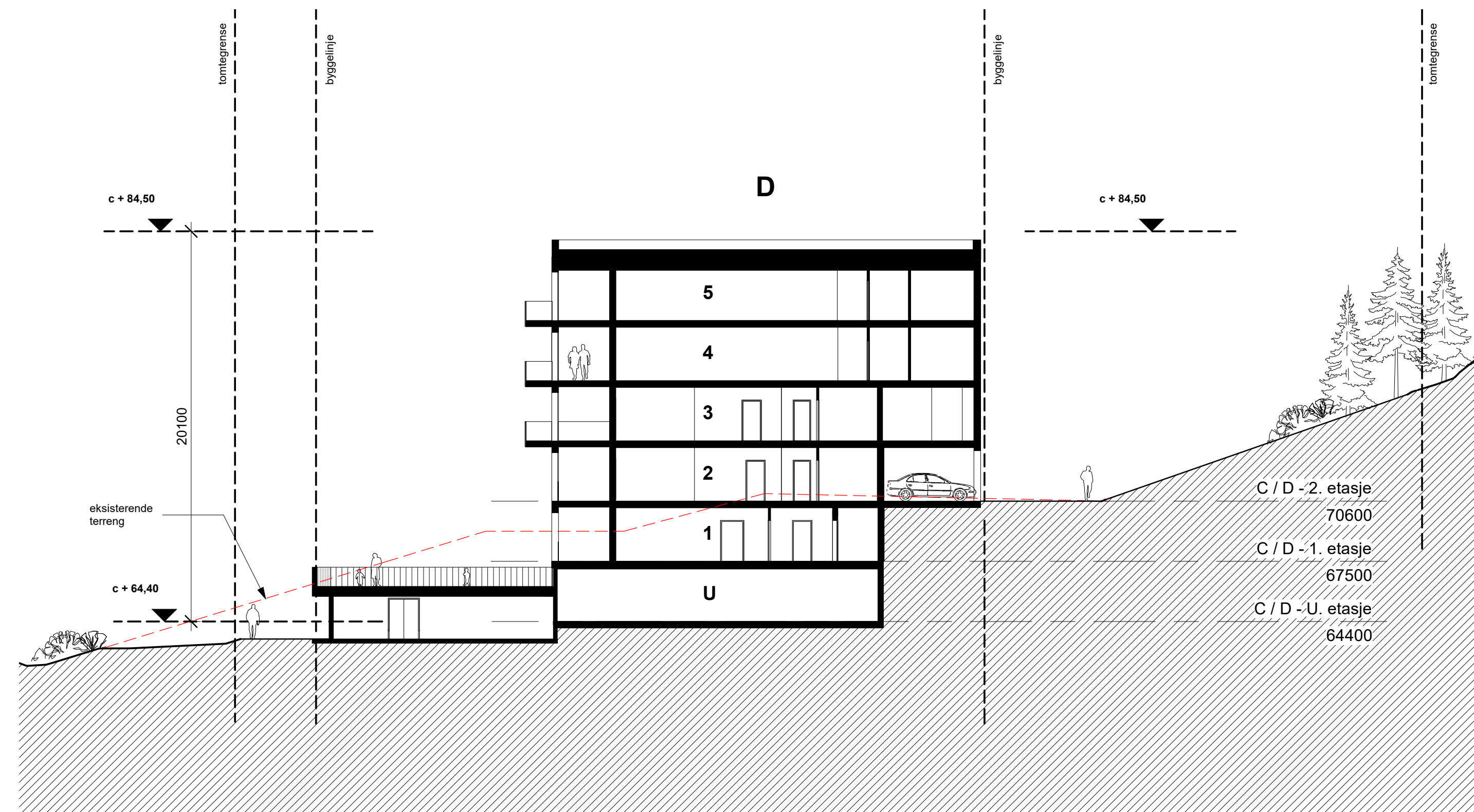
2 Snitt D-D 1 : 200
