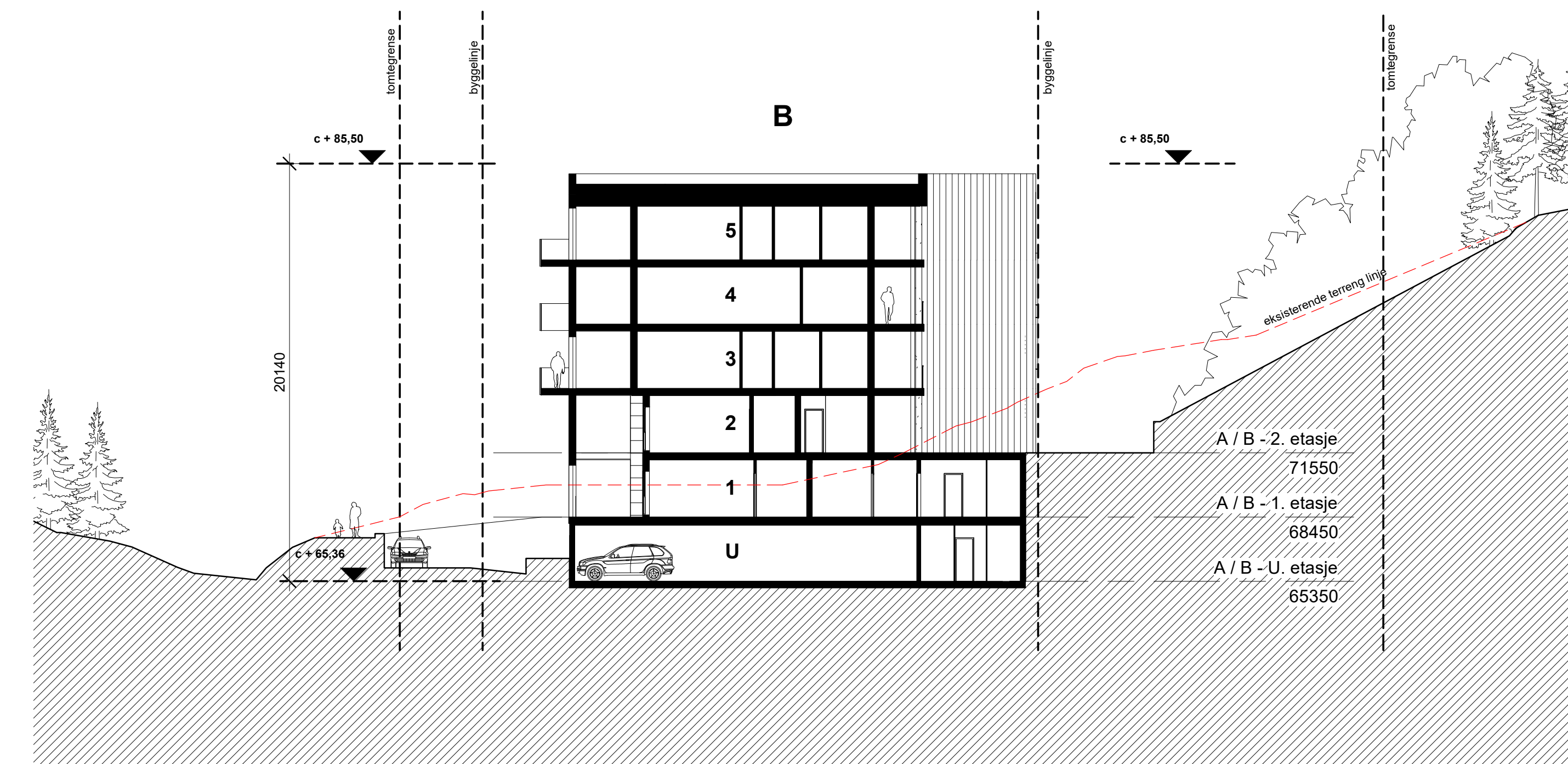
2 Snitt B-B 1 : 200
