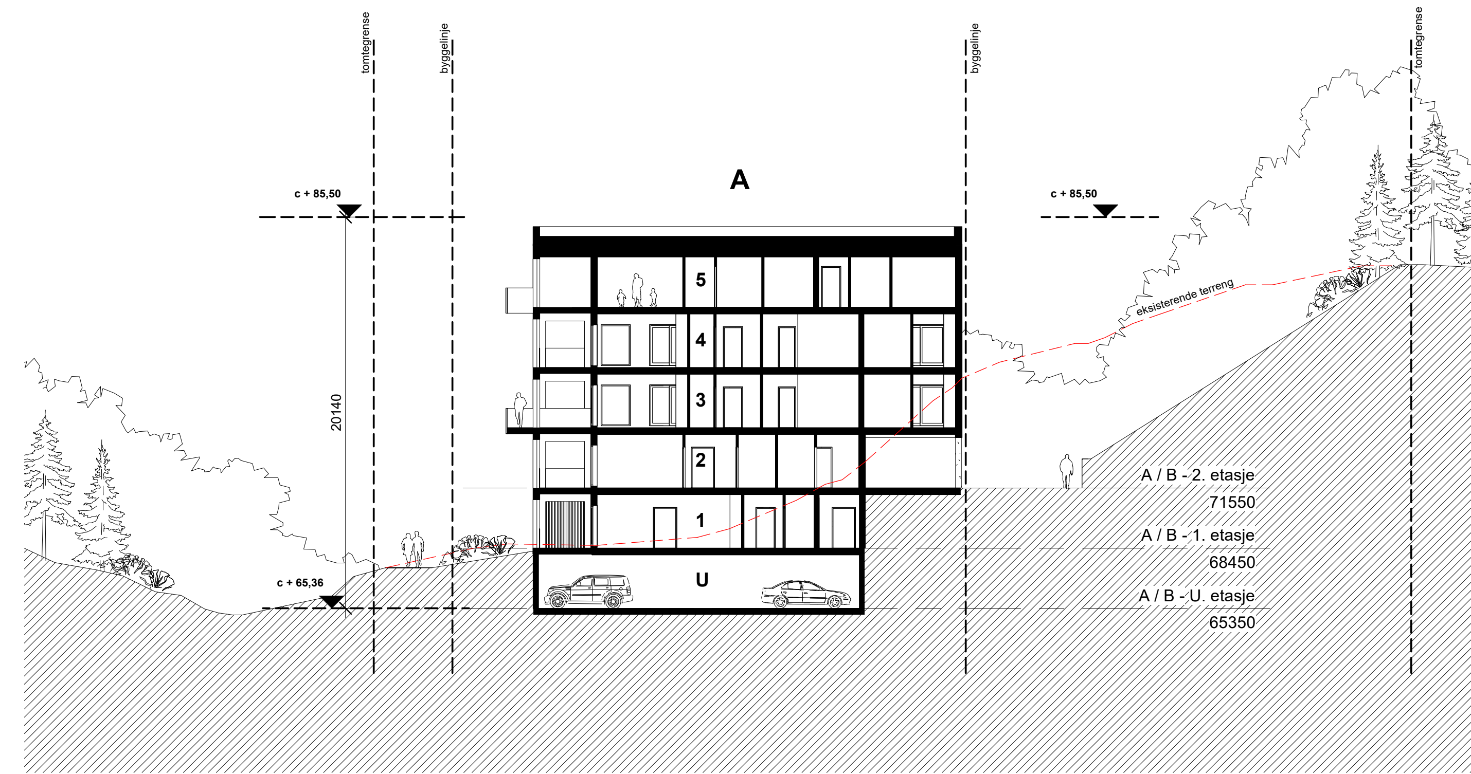
1 Snitt A-A 1 : 200
