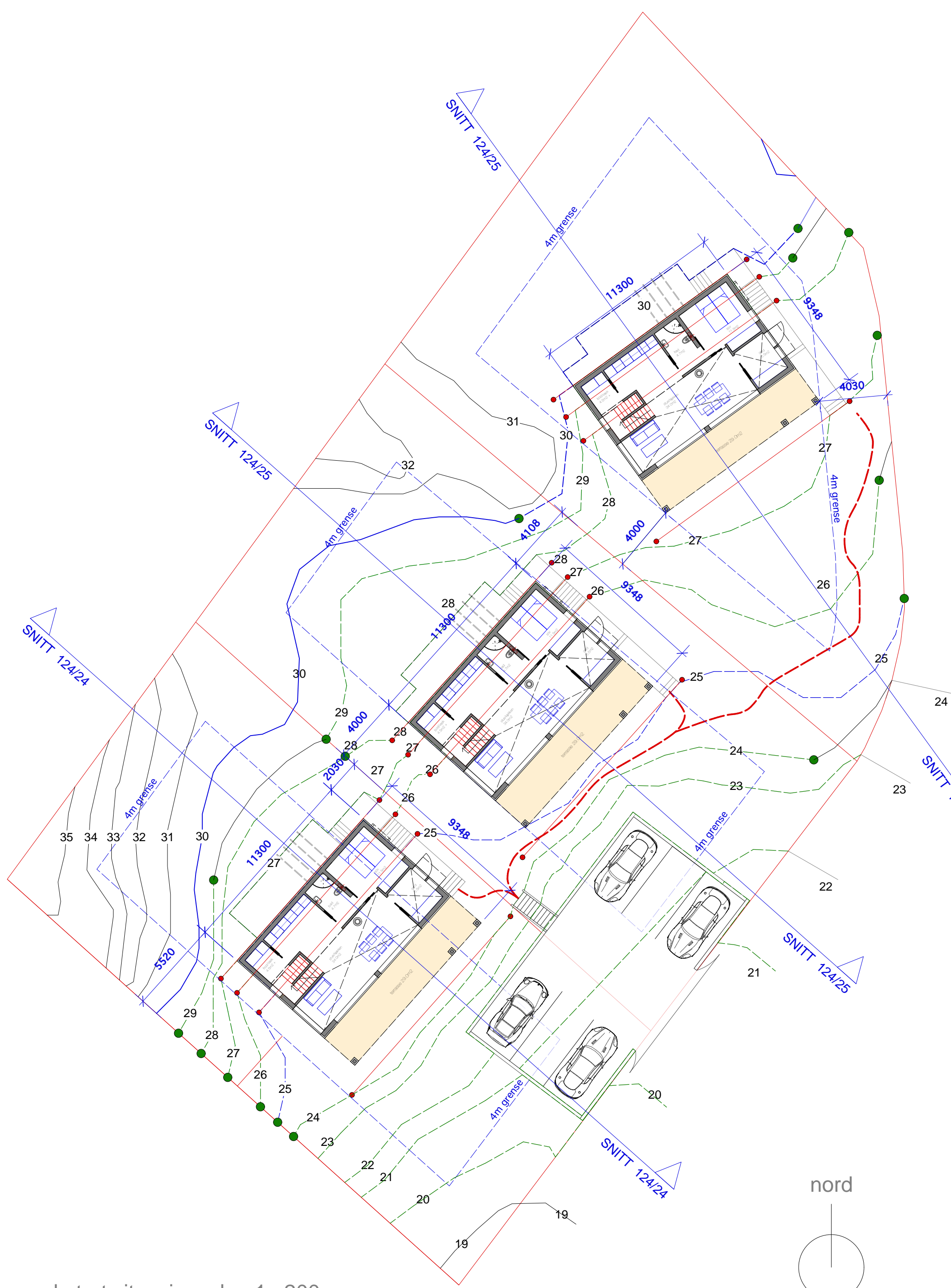
kotert situasjonsplan 1 : 200
