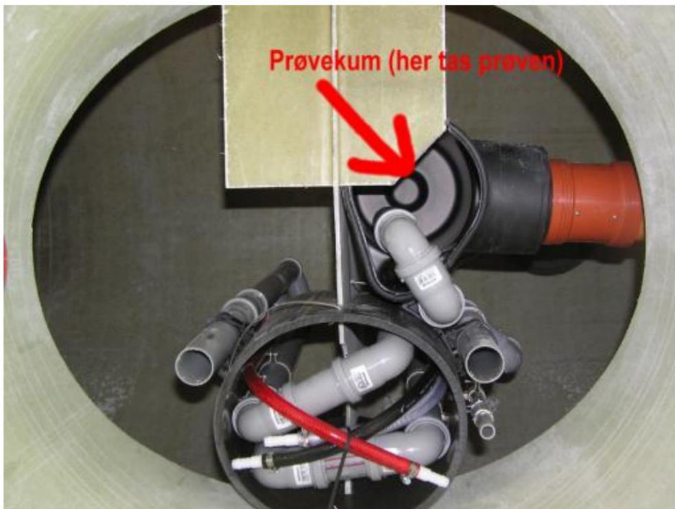
Skisse av Klaro minirensanlegg glassfiber med montert prøvetakingskum.
