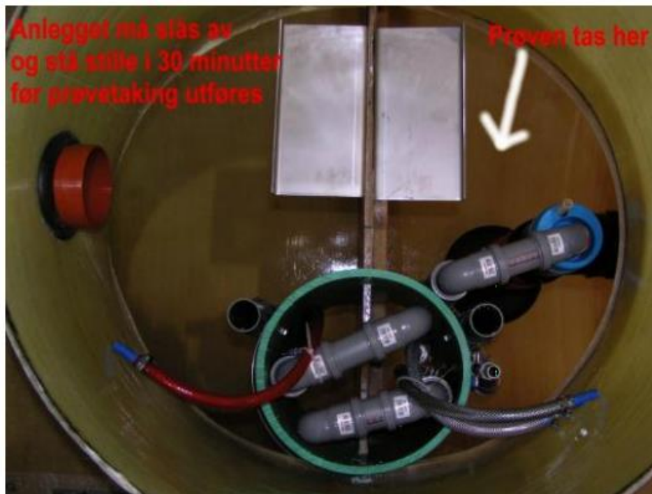
Skisse av KLAO Minirensanlegg- Glassfiber.
