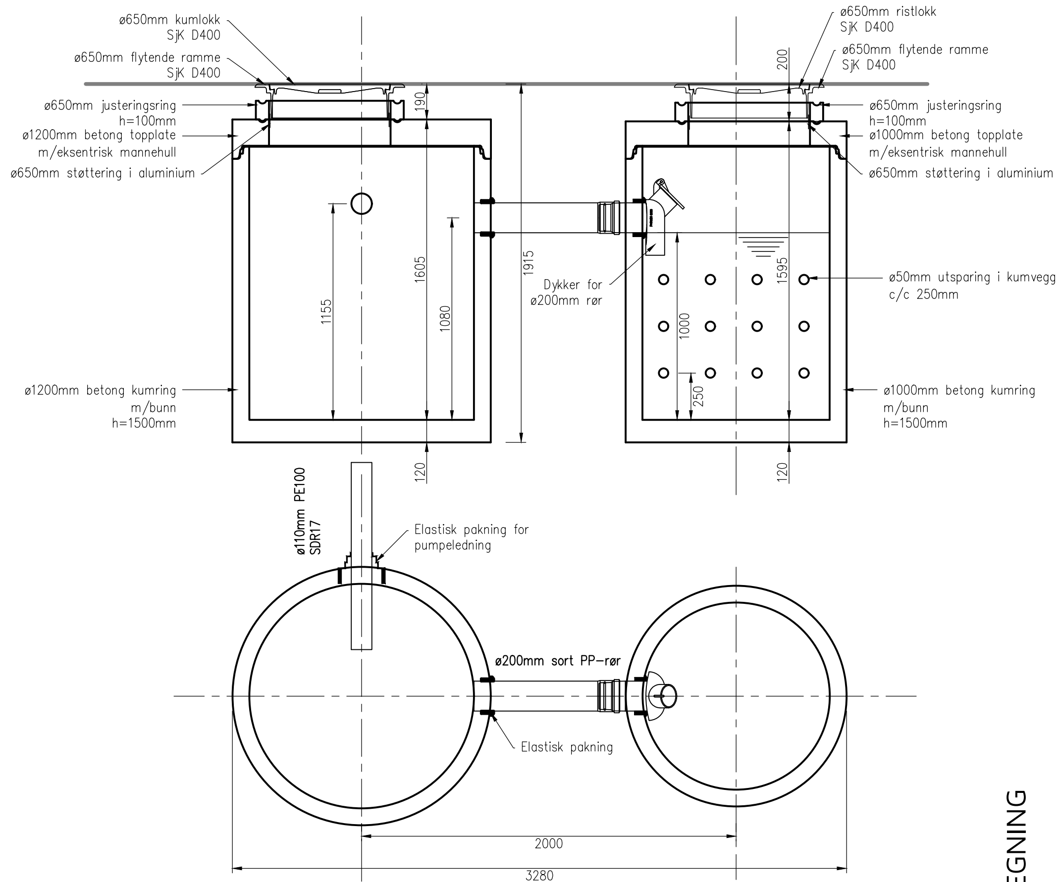
PLAN OG SNITT DRENS- OG PUMPEKUM M=1:20
