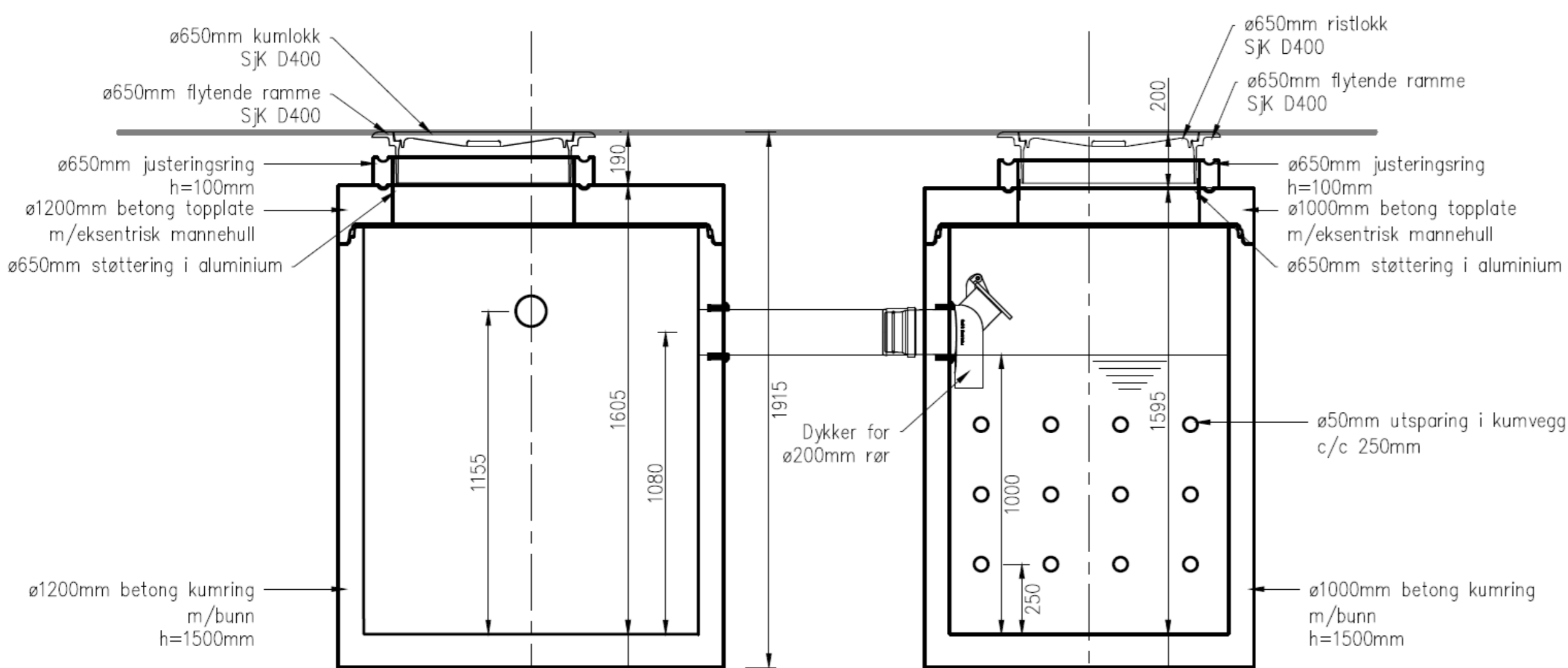
PRINSIPTEGNING PUMPE- OG DRENSKUM, SE OGSÅ DETALJTEGNING GH10
