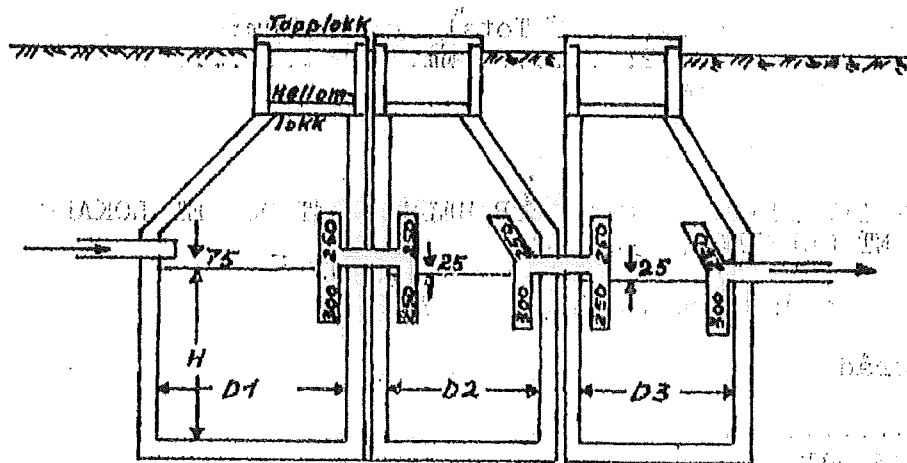
Fig. 5. Prinsipiell skisse av systemet. (Alle mål er minimumsavstander)
