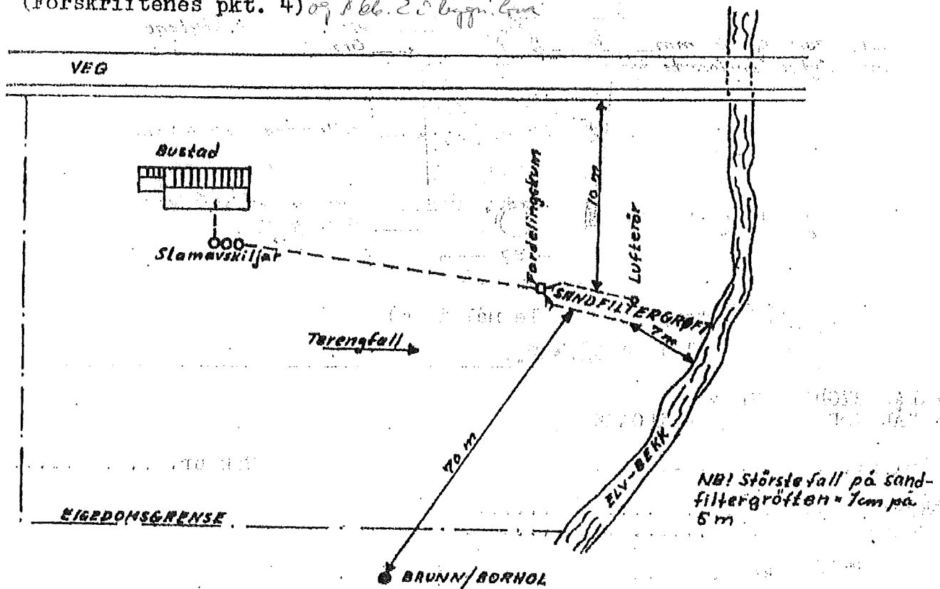
Fig. 5. Prinsipiell skisse av systemet. (Alle mål er minimumsavstander)
