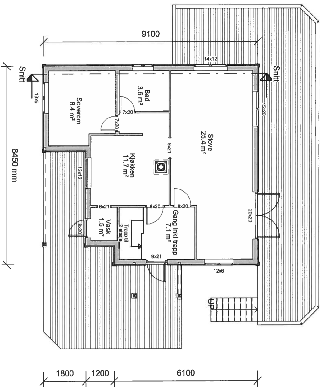
1 Etasje 1 : 100
