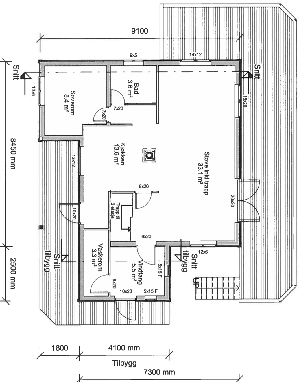
1 Etasje 1 : 100
