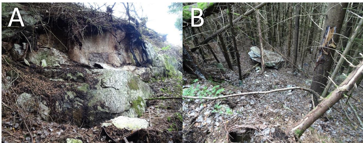
Figur 4. A) Løsnakeområde for relativt ferskt steinsprang. Merk de mørke røttene som vokser på utsiden av det ferske bruddet. Bildet er tatt mot øst. B) Steinsprangblokk på om lag 2 m 3 . Bildet er tatt mot sørvest.
