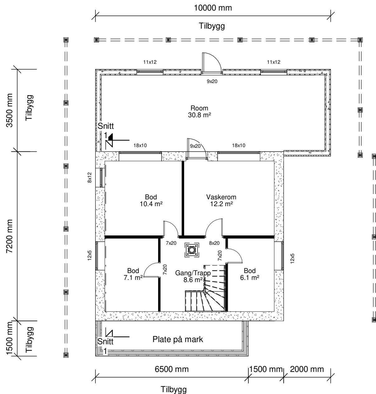
0 KJELLER 1 : 100
