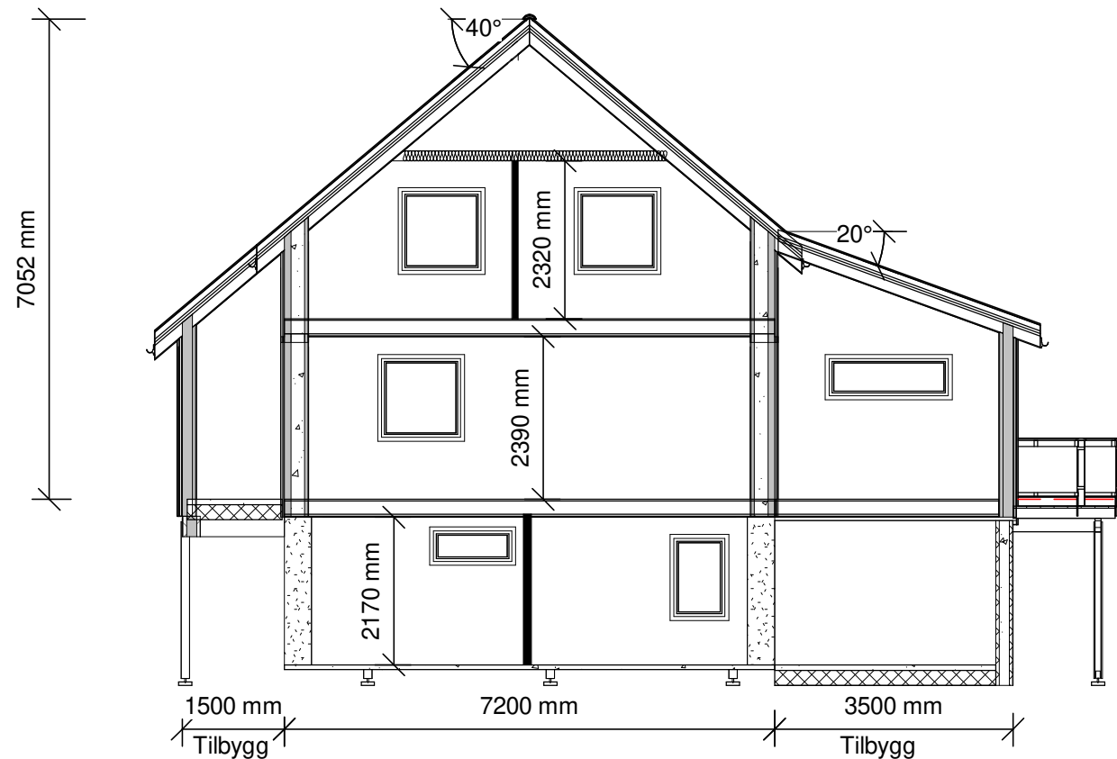
Snitt 1 1 : 100
