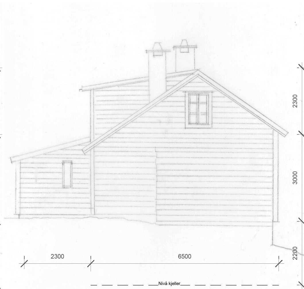
FASADE NORD- ENDRET
