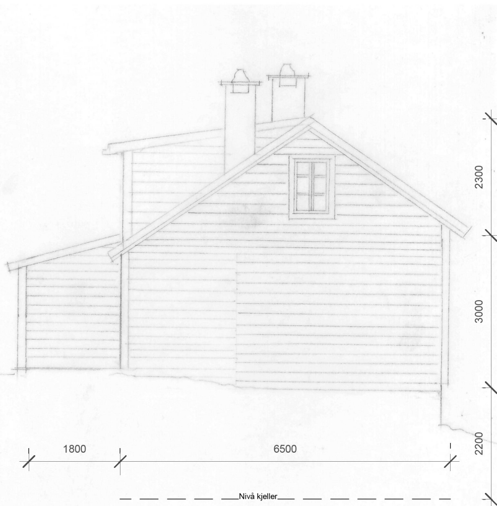
FASADE NORD- EKSISTERENDE
