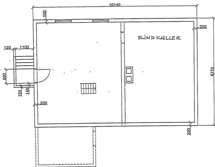
PLAN KJELLER
