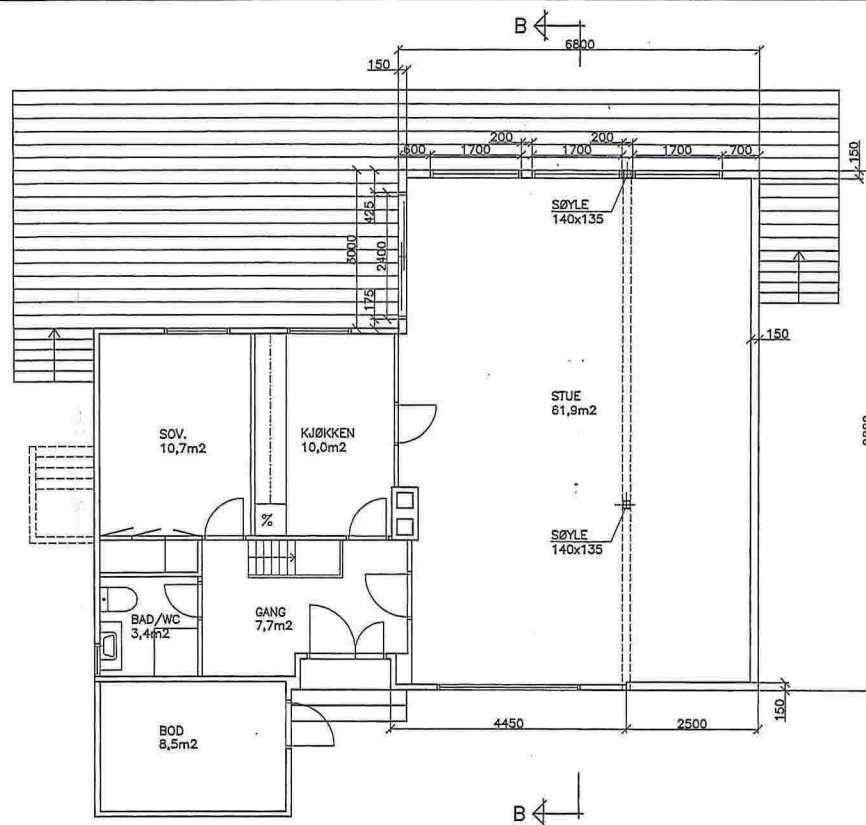
PLAN 1.ETASJE
