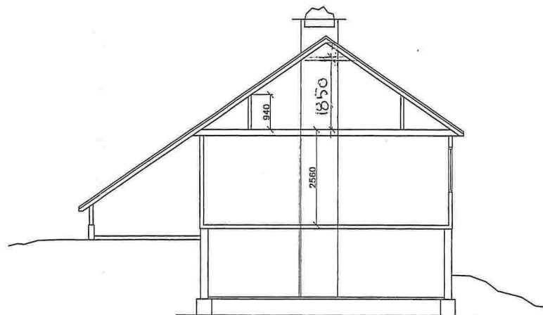
SNITT A-A
