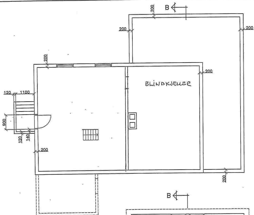
PLAN KJELLER
