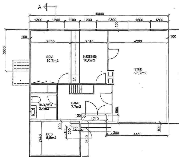
PLAN 1.ETASJE
