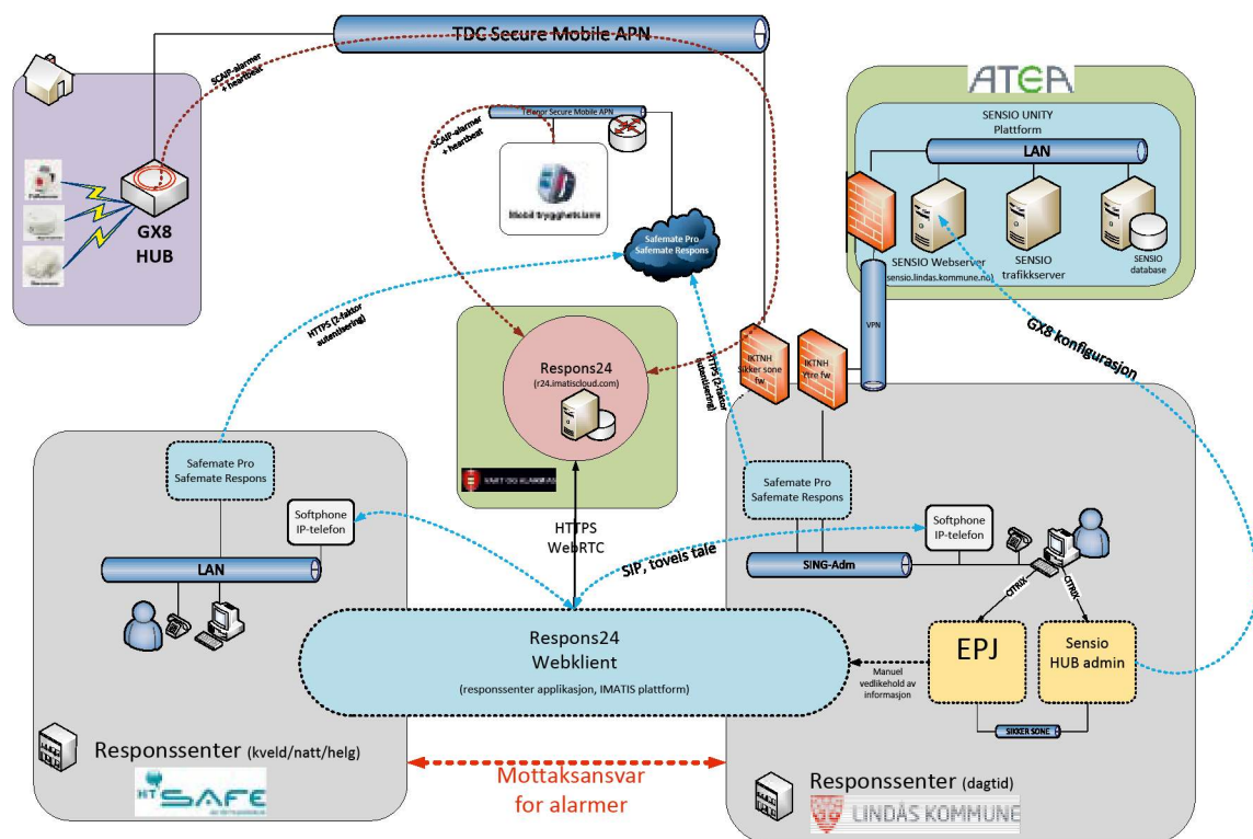
Figur 2. Skisse av den tekniske løysinga. Brukarens heim er vist øvre venstre hjørna i figuren, sensorane i heimen saman med den mobile tryggingssentralen er teknologi som brukar ser.
