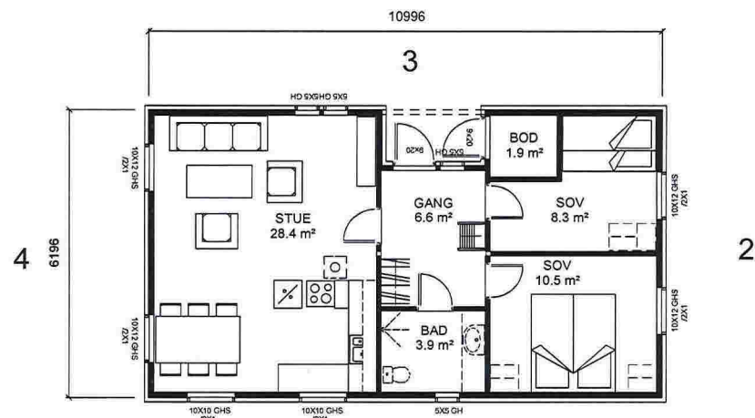
HOVEDPLAN 1
