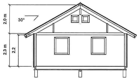
TYPISK SNITT VED HEMS
