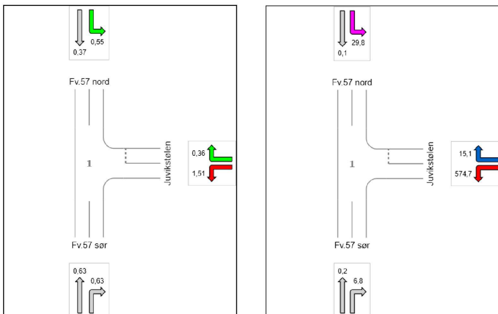
Figur 3. Belastningsgrad og forsinkelser pr. kjøretøy (sek), alternativ 1, 800 boliger.
