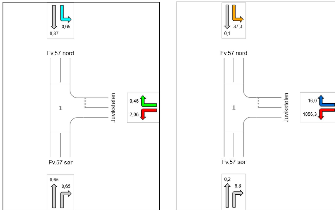
Figur 4. Belastningsgrad og forsinkelser pr. kjøretøysklasse (kjf. (sek)), alternativ 2, 1500 boliger.
