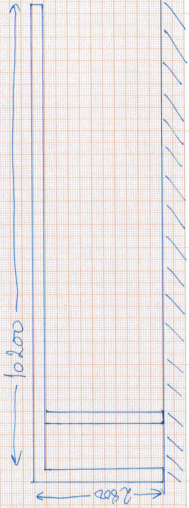
snitt side
