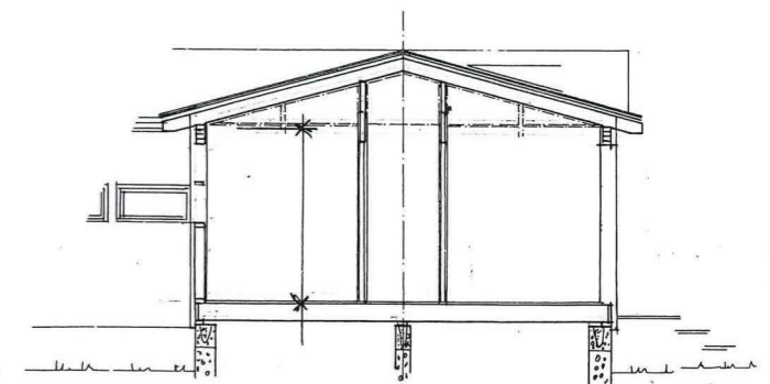
SNITT - tilbygg
