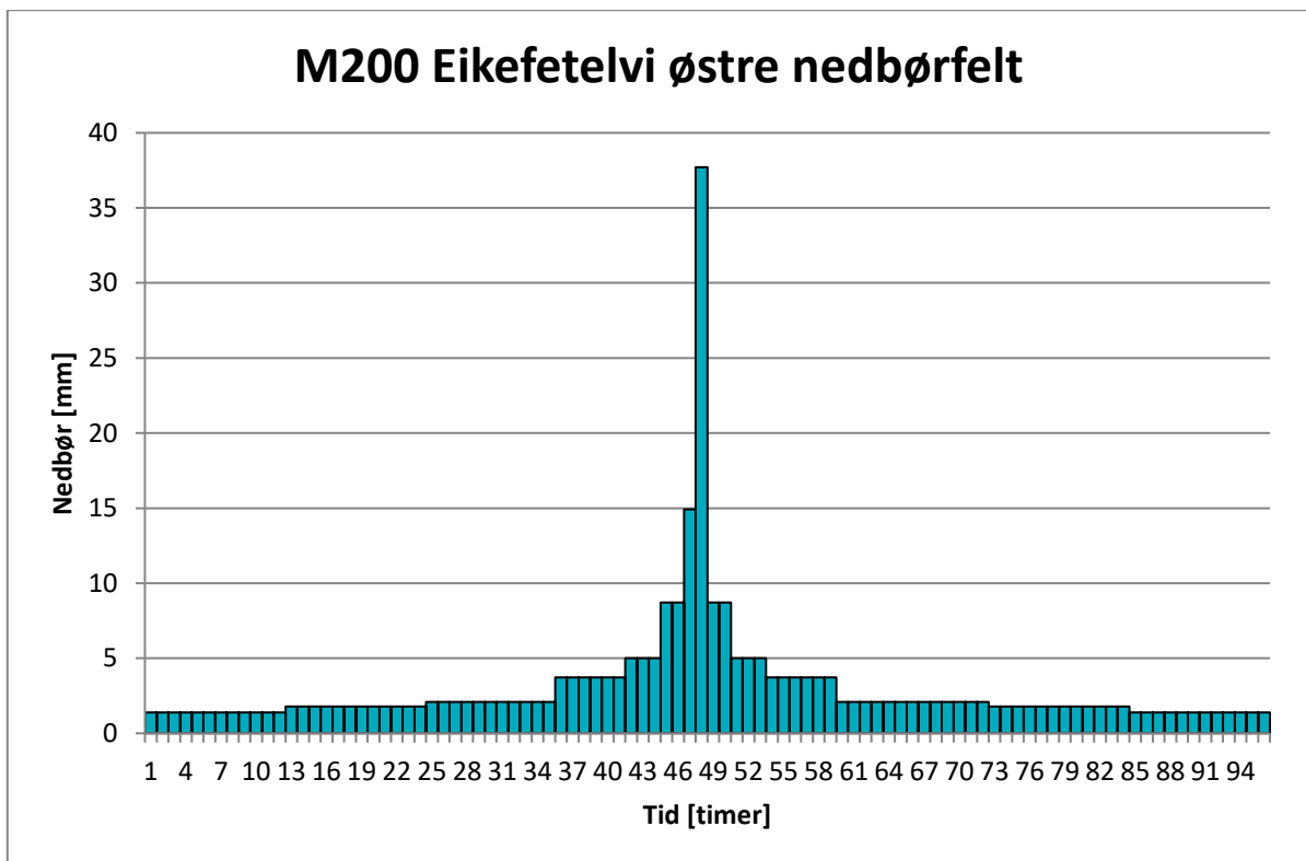
Figur 0-3 Syntetisk konstruert nedbørforløp med 200 års gjentakintervall
