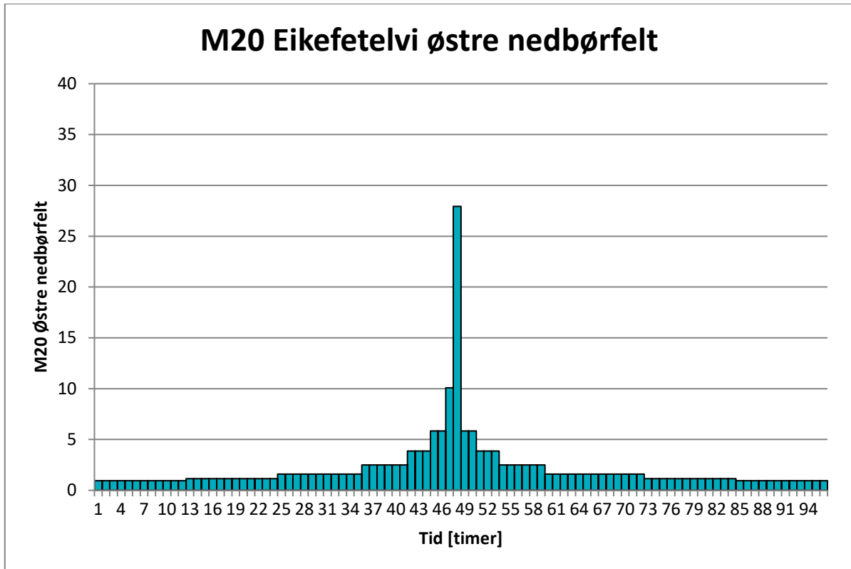
Figur 0-2 Syntetisk konstruert nedbørforløp med 20 års gjentakintervall
