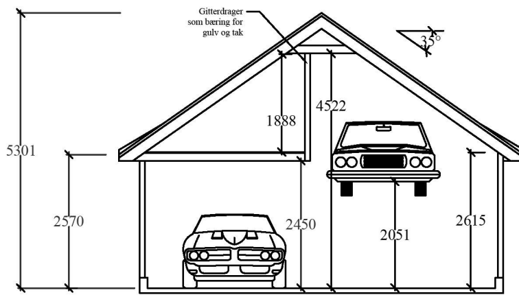
Snitt B-B
