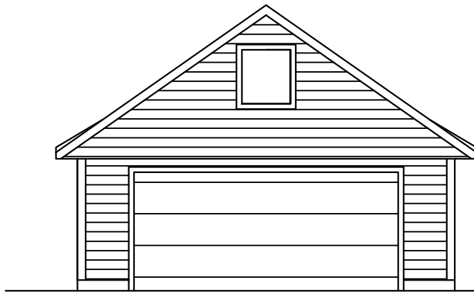
Fasade Sør-Vest
