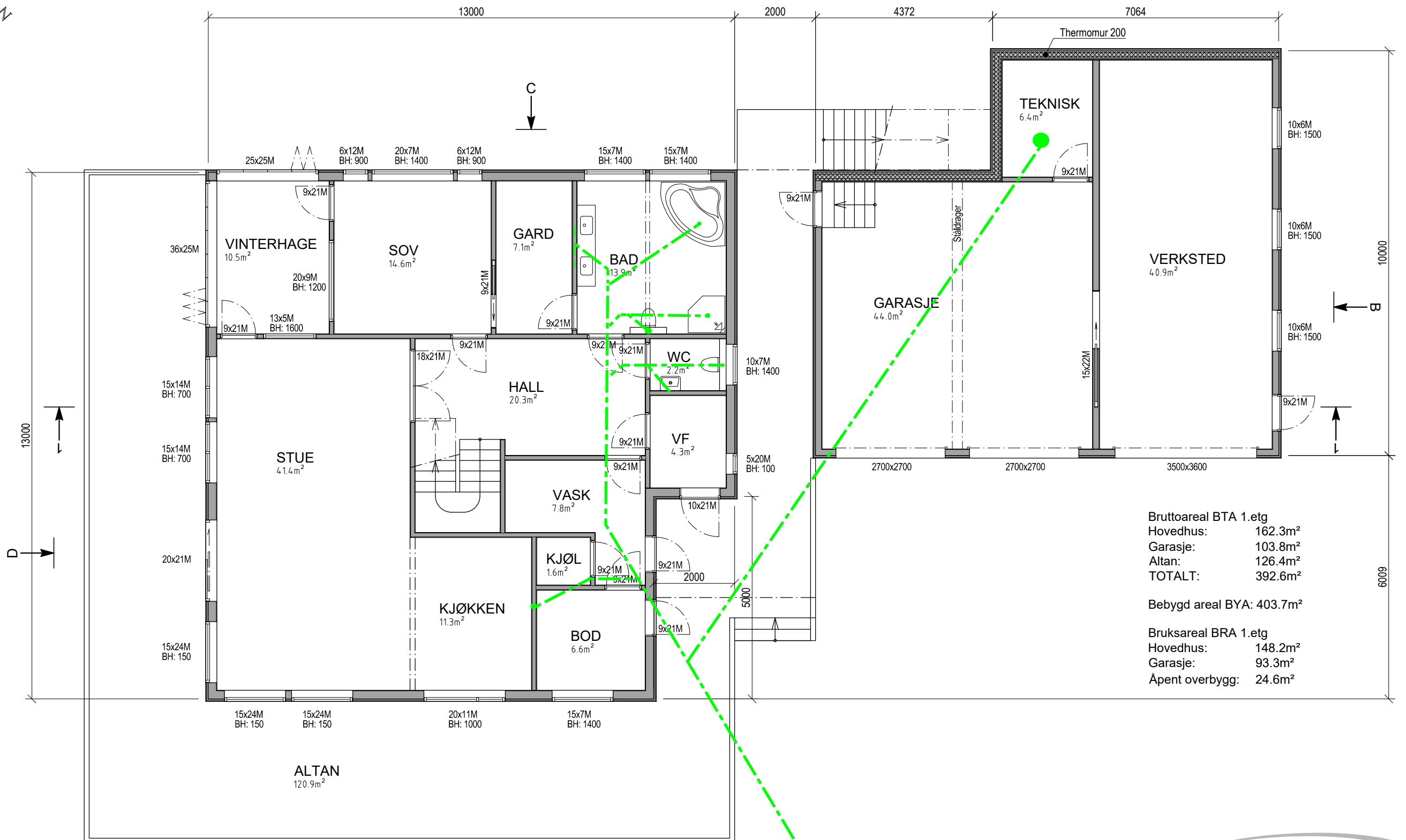
PLAN 1.ETG
