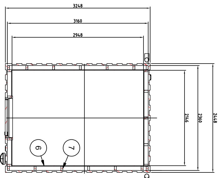
Sektion A-A
