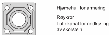
Fig. 435 Eksempler på skorsteins-elementer
