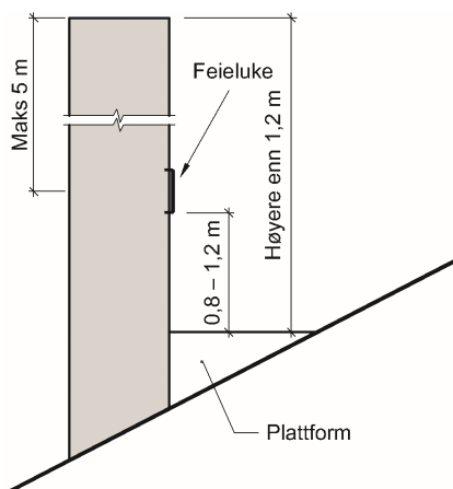
Fig. 61 b Krav til mål ved feiing via feieluke plassert over tak
