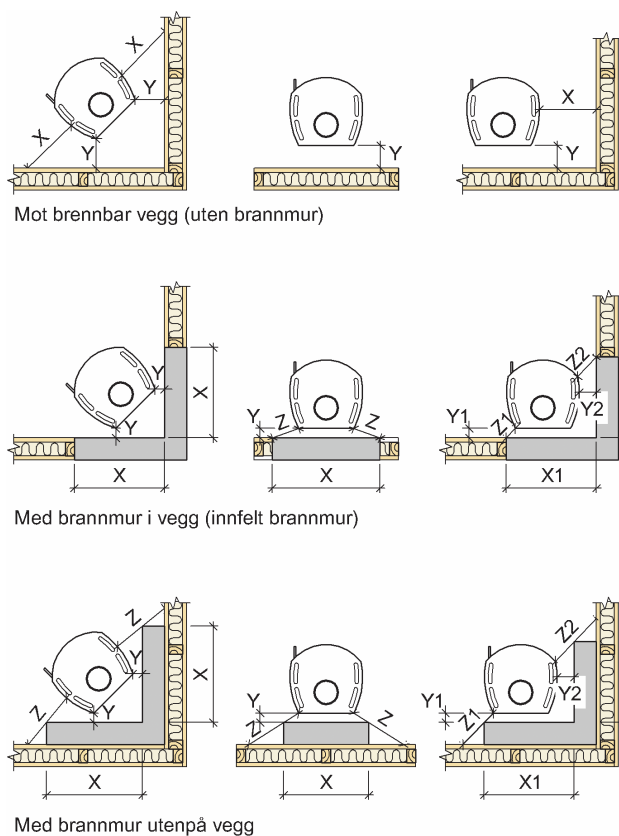
Fig. 33 Eksempler på monteringsmål fra produsent
