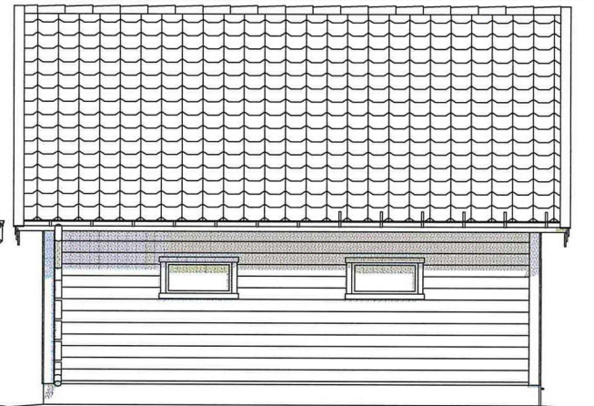
Fasade 4 1:100
