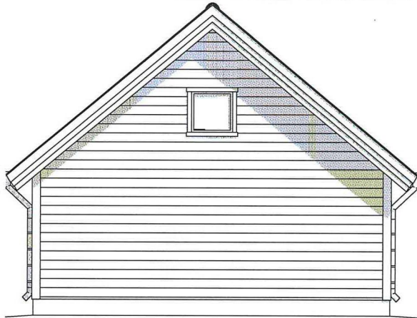
Fasade 2 1:100
