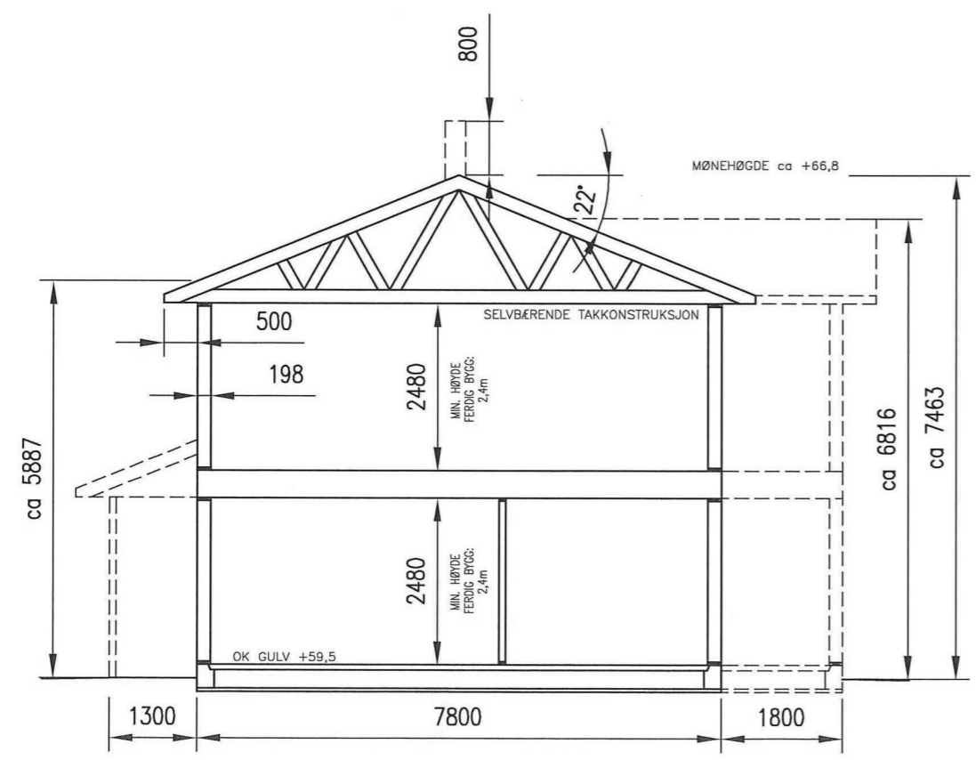
TYPISK SNITT
