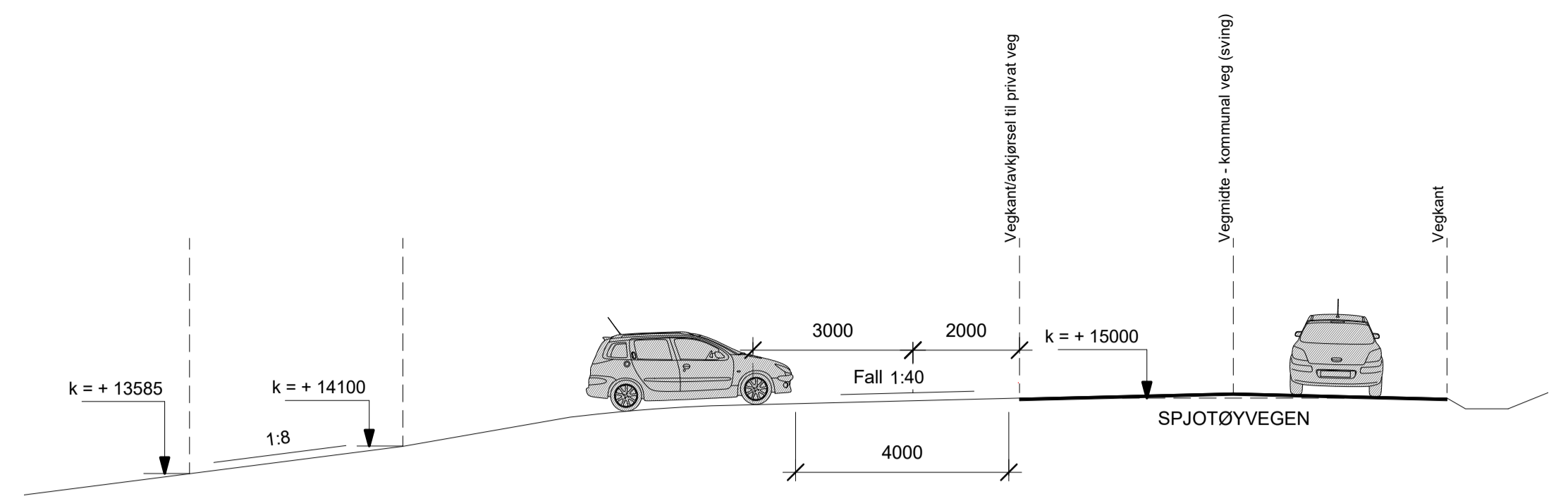
LENGDEPROFIL FOR AVKJØRSEL, MÅLESTOKK 1:100 VED ARKSTR. A1
