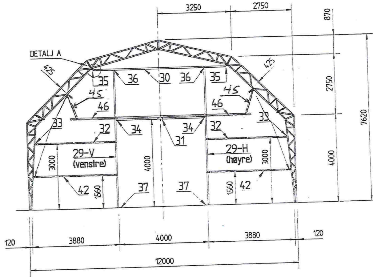
OPPRISS GAVLFORGITRING 1:100
