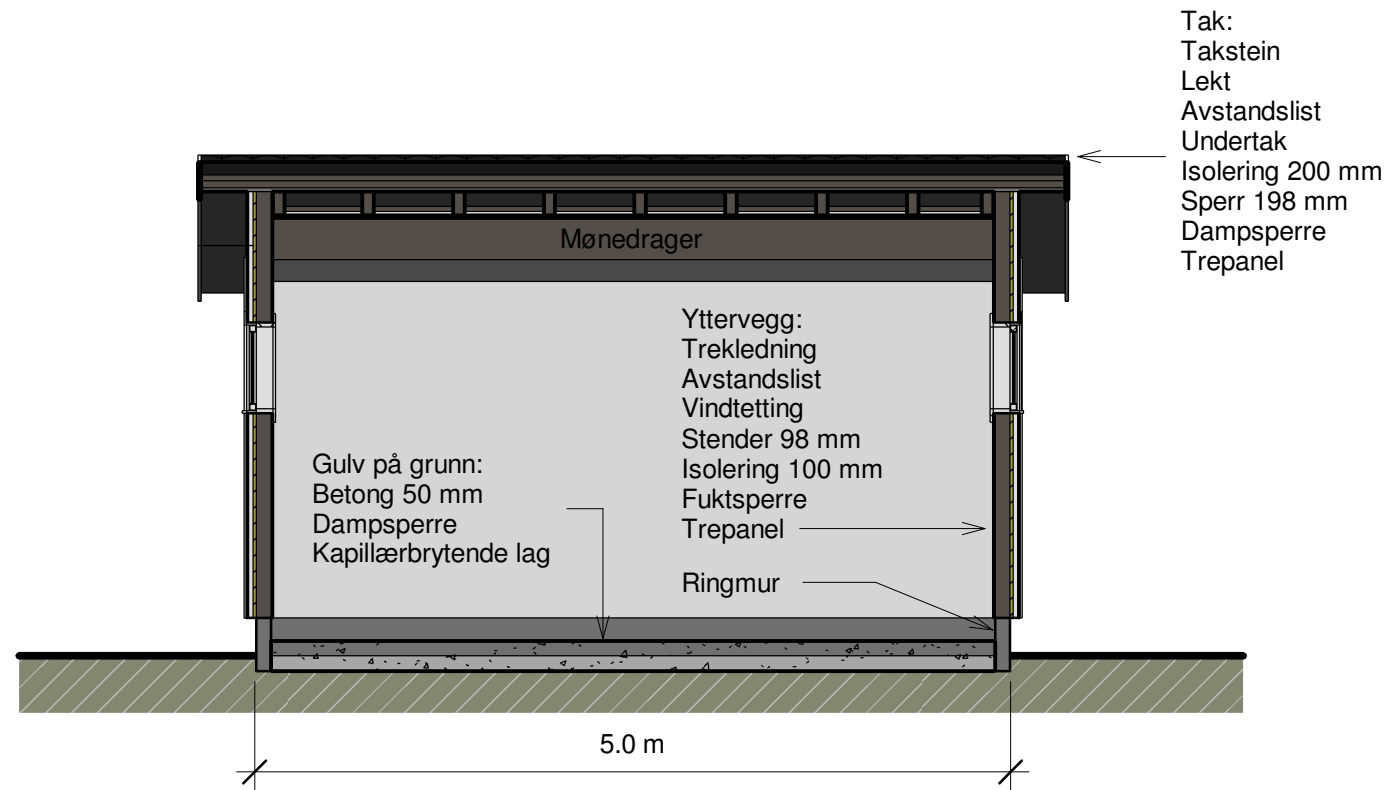
LANGSNITT
