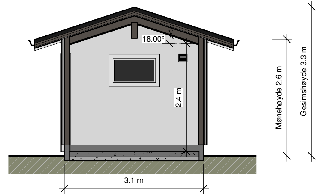
TVERRSNITT
