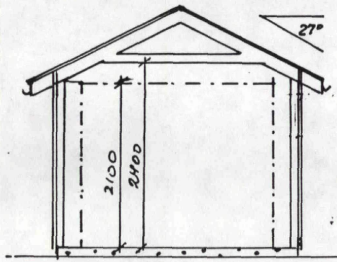
SNITT.
