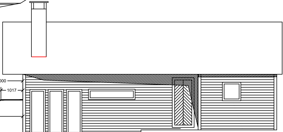
PROFIL AKSE 2
