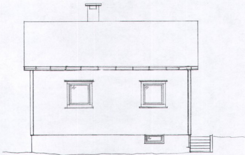
FASADE VEST
