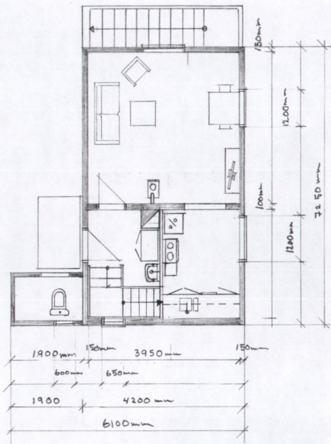
PLANS 1. ETG.
