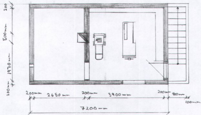
PLAN KJELLER
