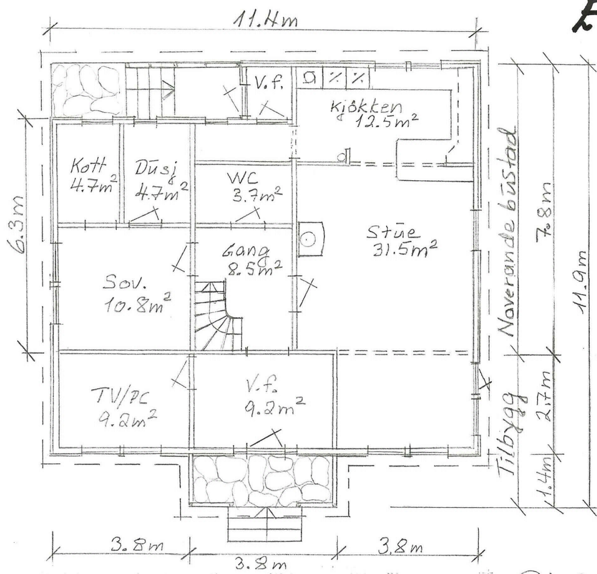
PLAN 1. ETG.
