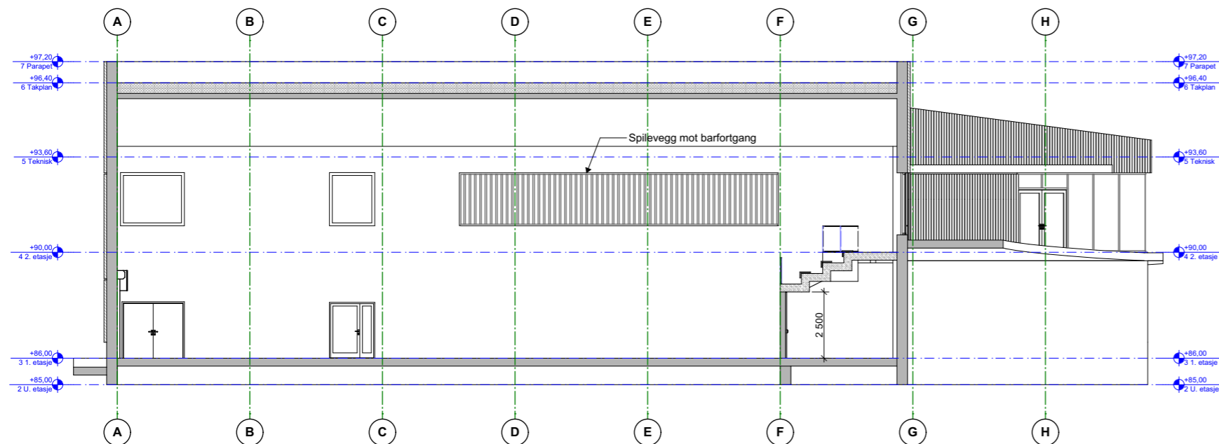
1:200 Snitt C
