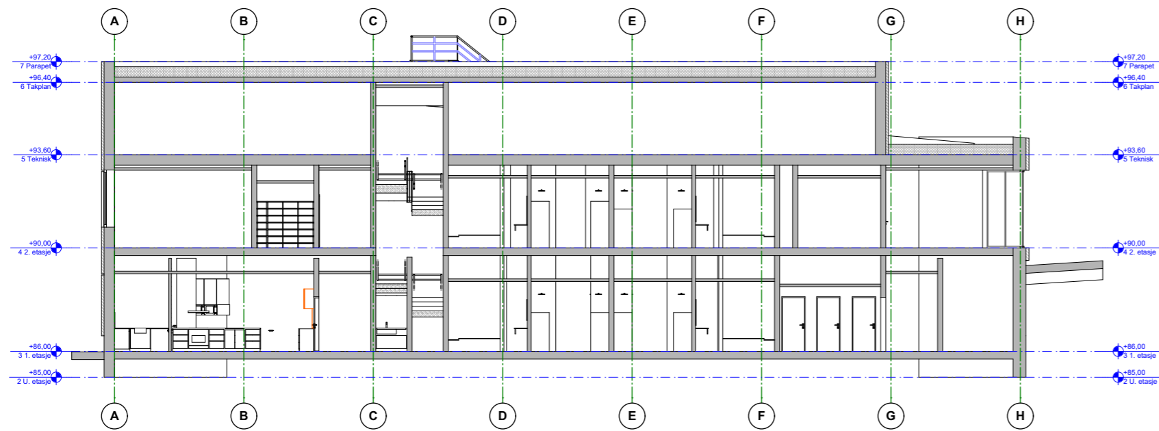
1:200 Snitt B
