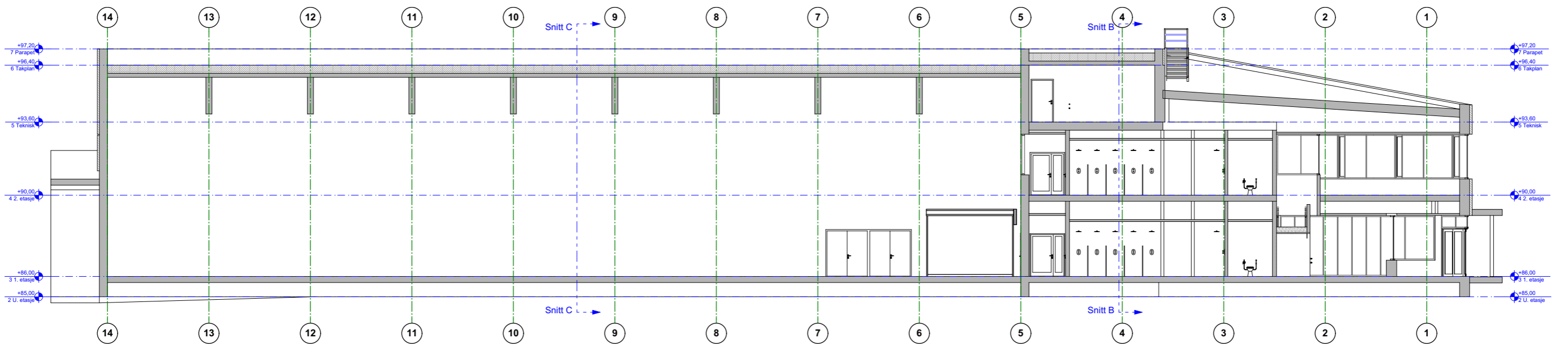
1:200 Snitt D
