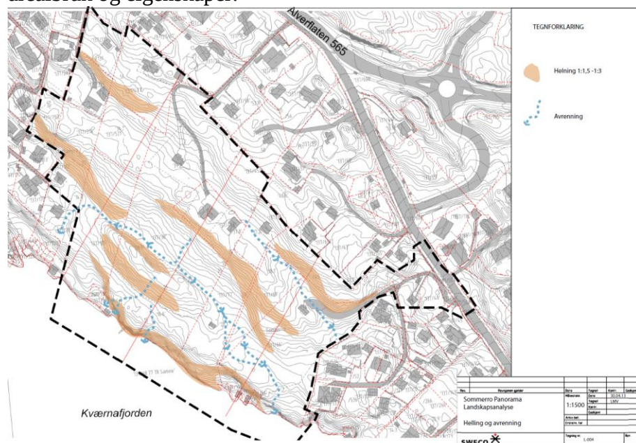
Bilde: Hellingsskart som viser helning 1:1,5 og 1:3 og avrenning. Kjelde Sweco
