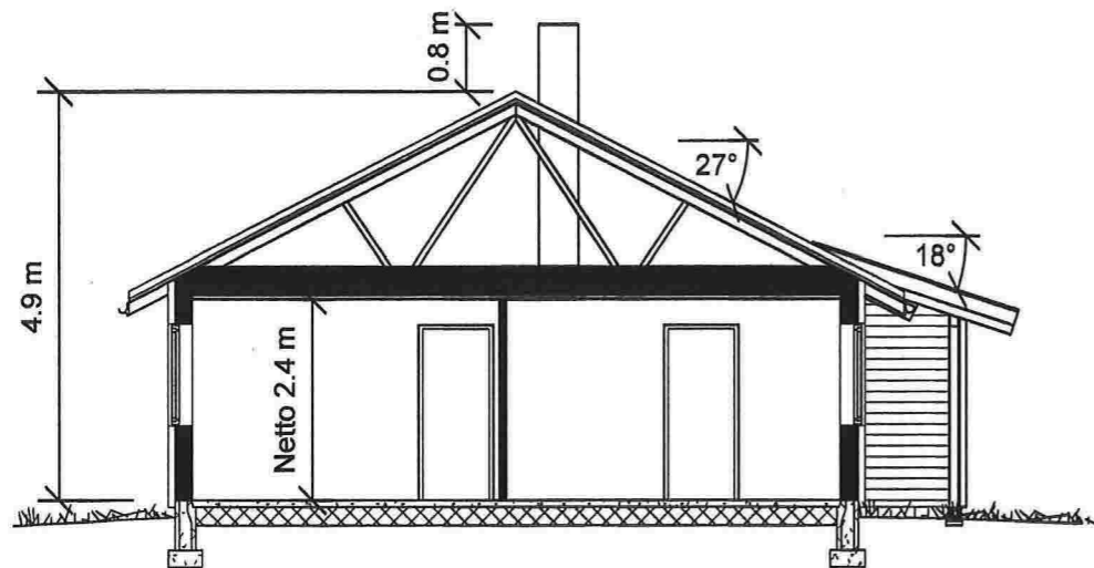
Snitt A-A
