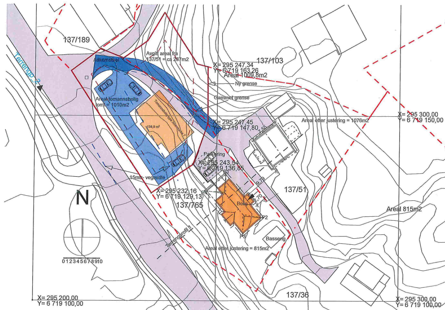
Situasjonskisse, 1:500
