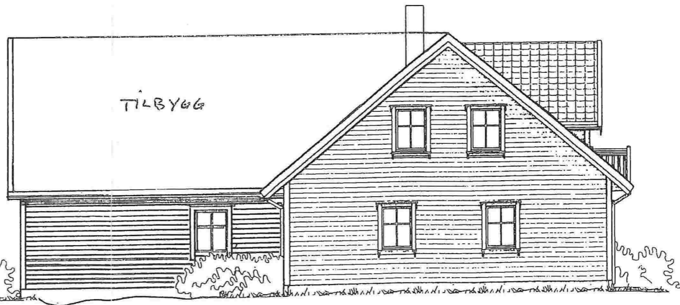
FASADE 4
